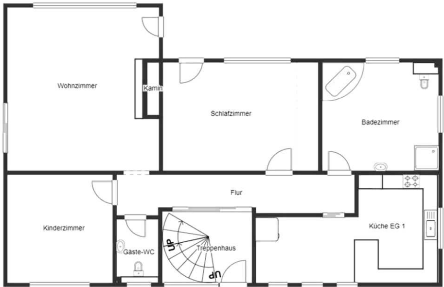
Grundriss Skizze EG
