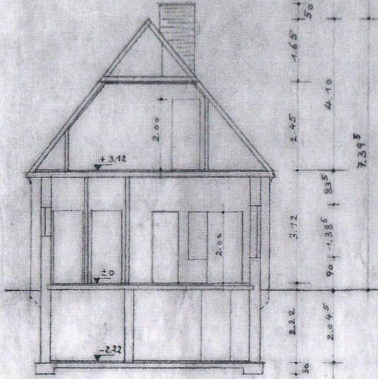
SCHNITT A-B
