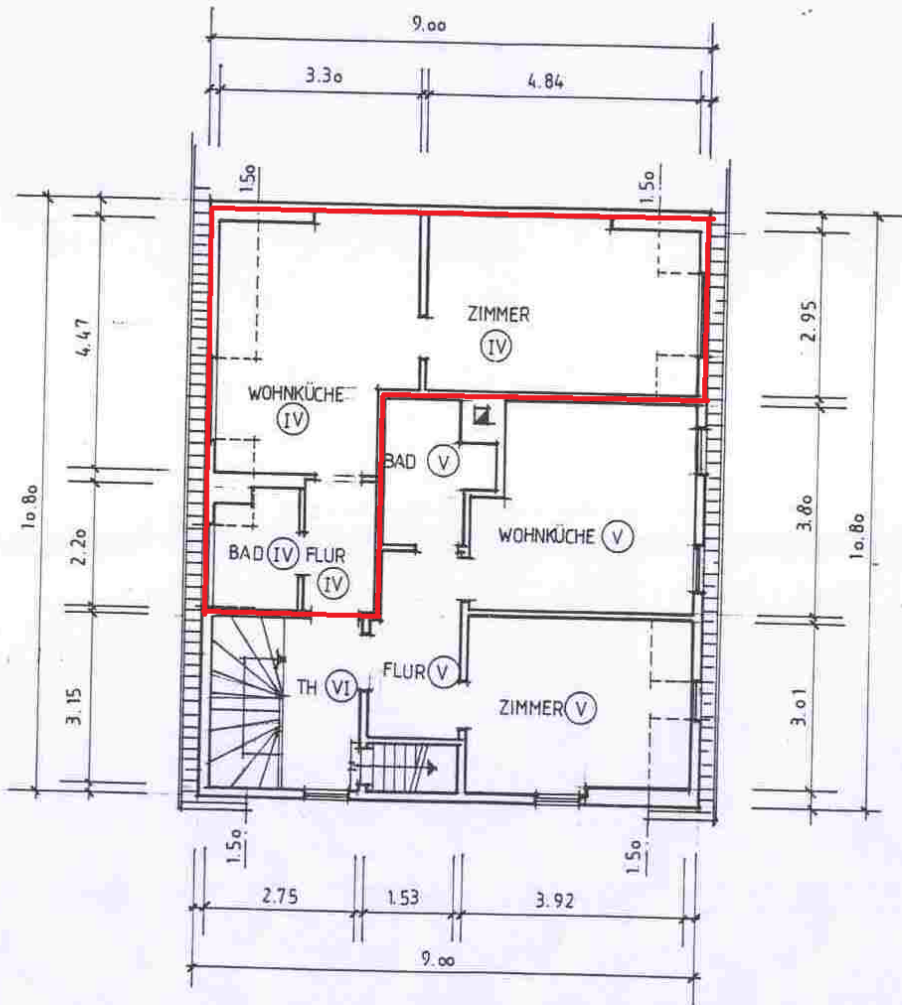
DACHGESCHOSS M 1:100
