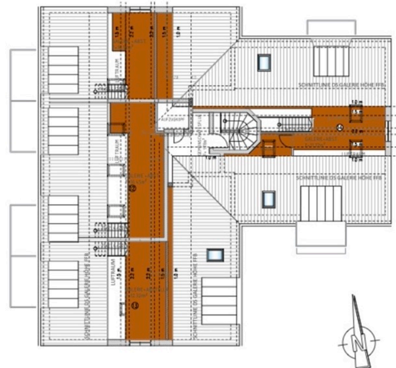
GRUNDRISS DS 1:100
