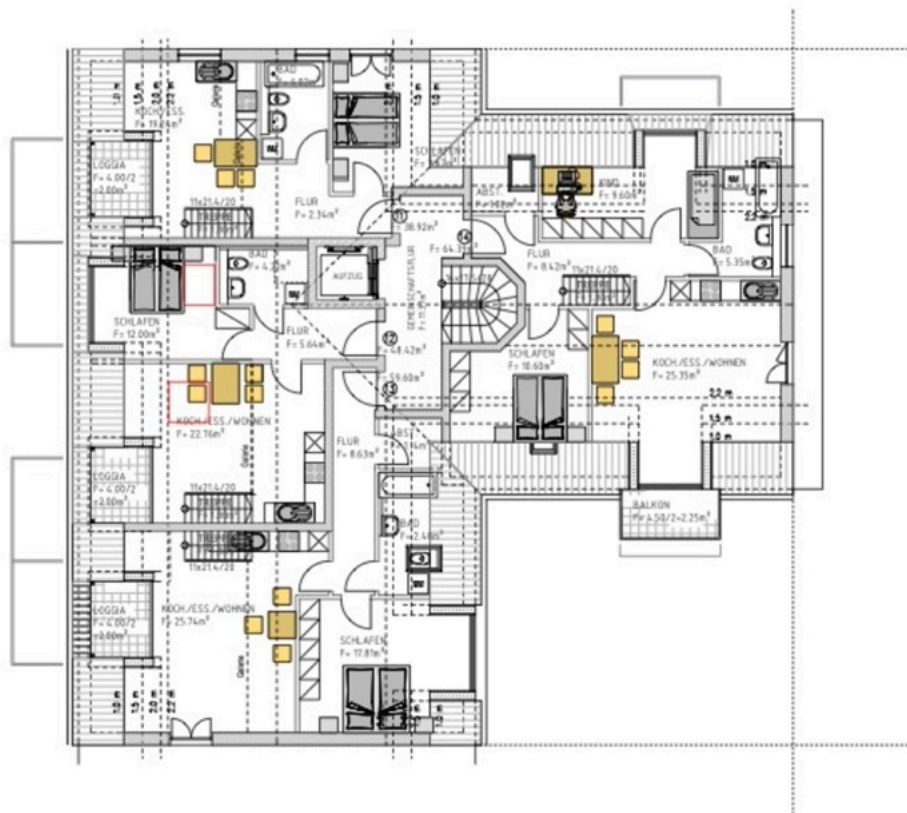
GRUNDRISS DG 1:100
