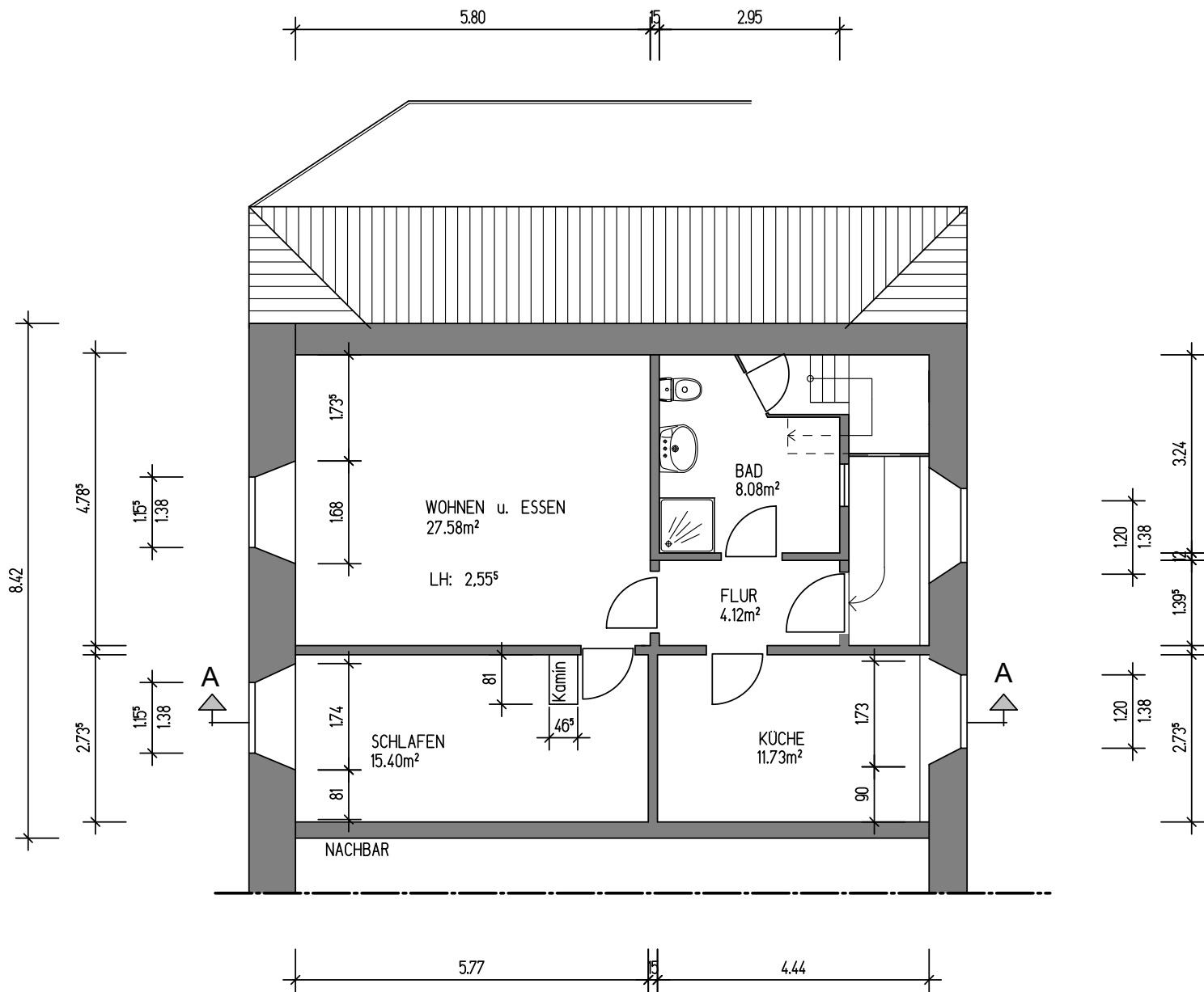
2. OBERGESCHOSS
