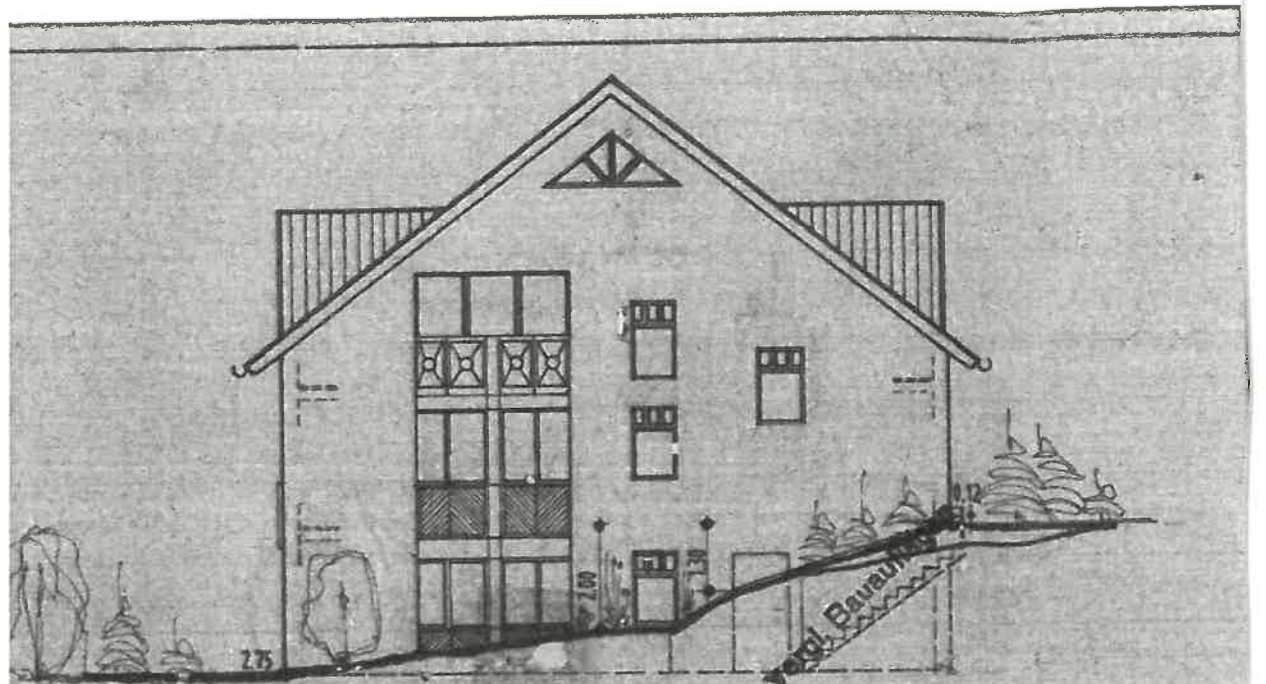
OSTANSICHT
