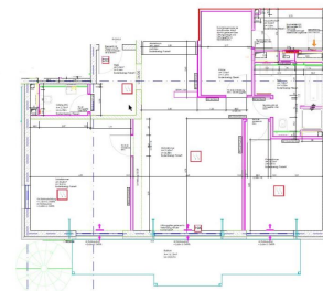
Grundriss
