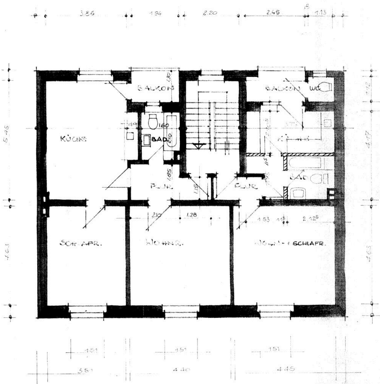
1.+2. OBERGESCHOSS
