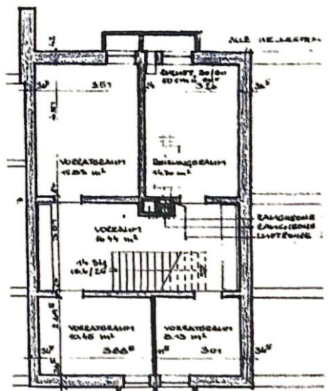
Kellergeschoss
