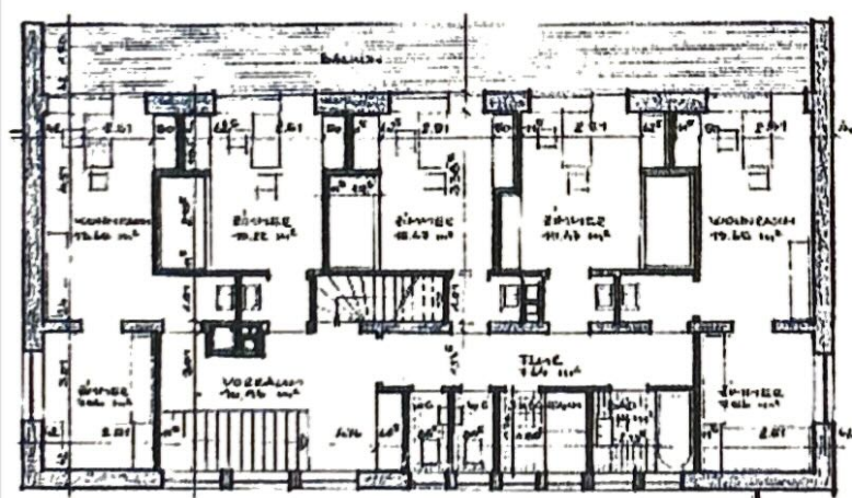
Obergeschoss
