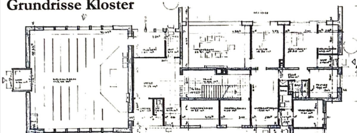
Erdgeschoss
