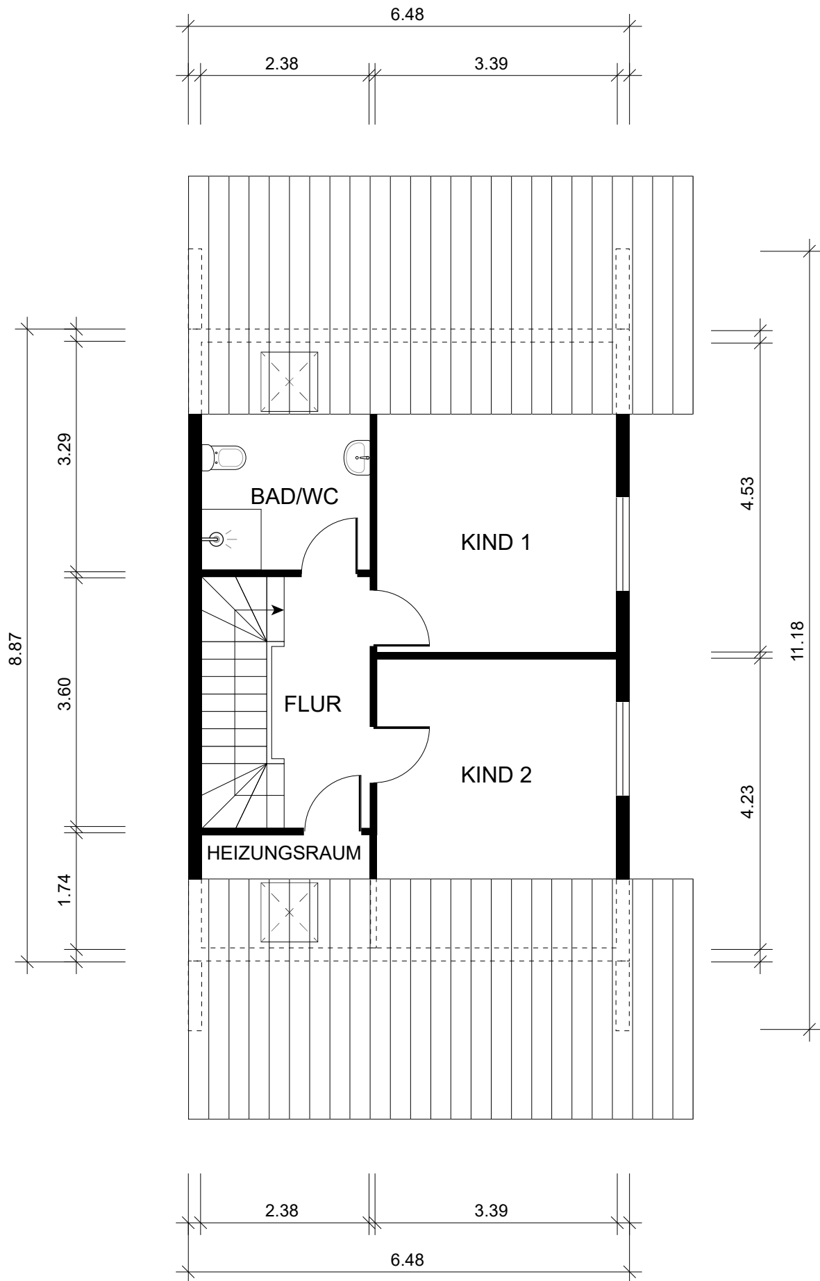
2. OBERGESCHOSS
