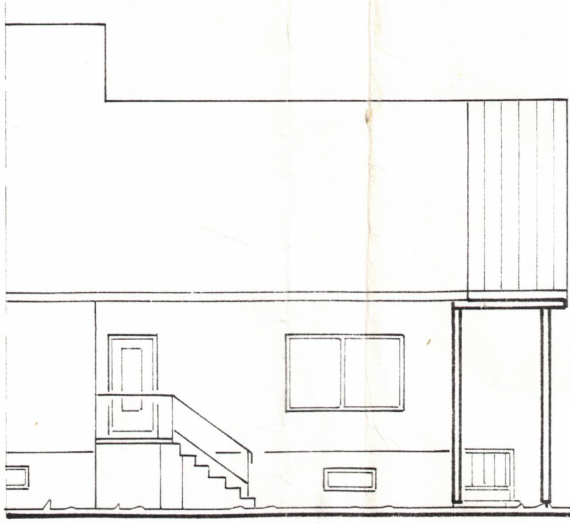
OST-ANSICHT
