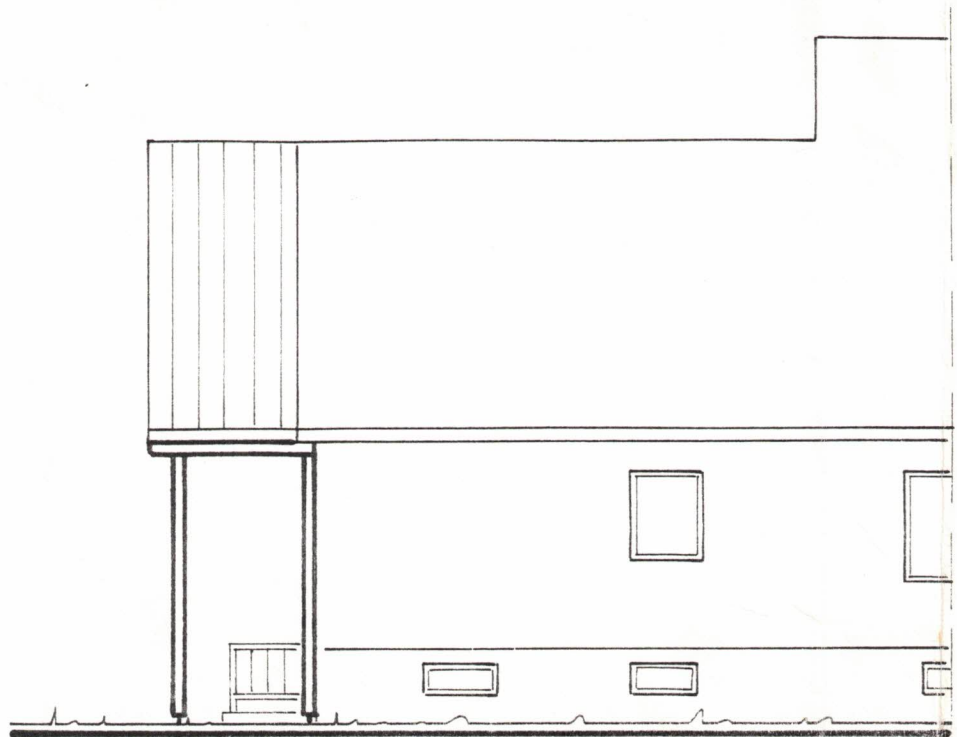
WEST-ANSICHT
