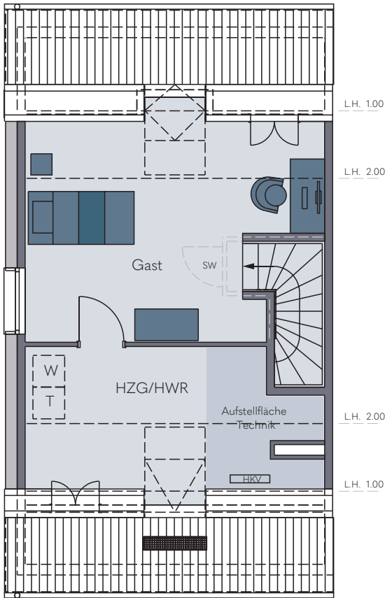
Dachgeschoss Reihenendhaus Nr. 1 Doppelhaushälfte Nr. 1
