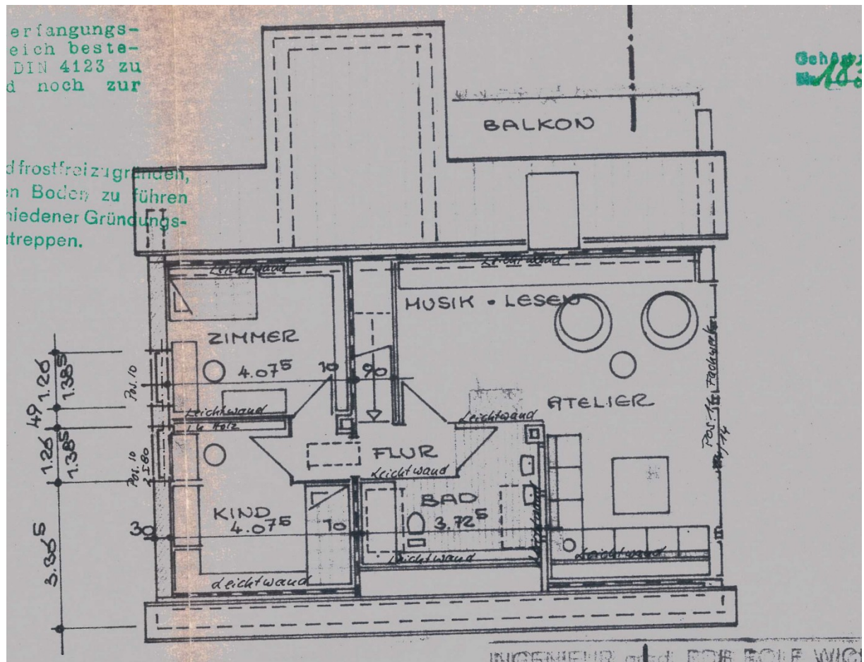
Grundrisszeichnung Dachgeschoss
