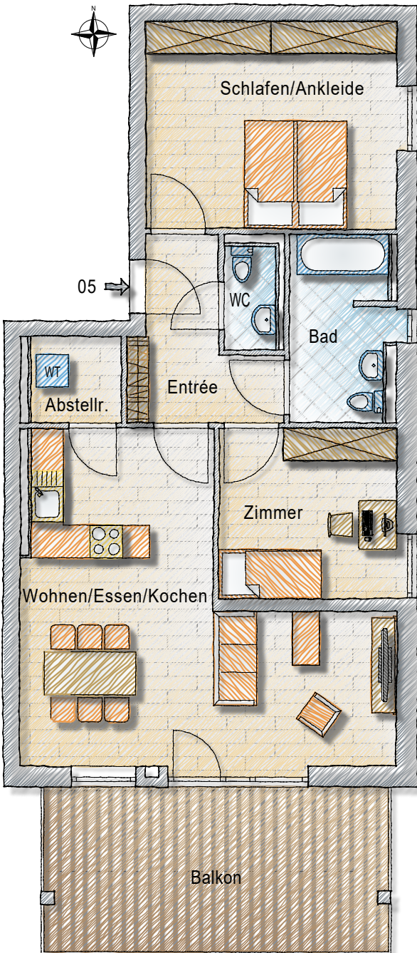
1 Obergeschoss
