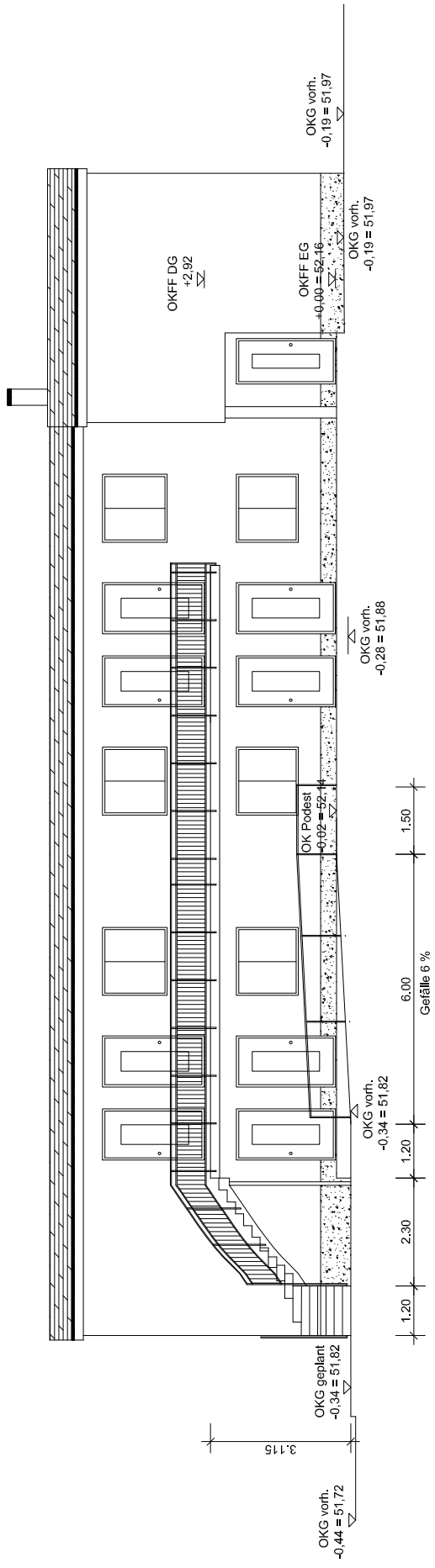
Ansicht NORD
