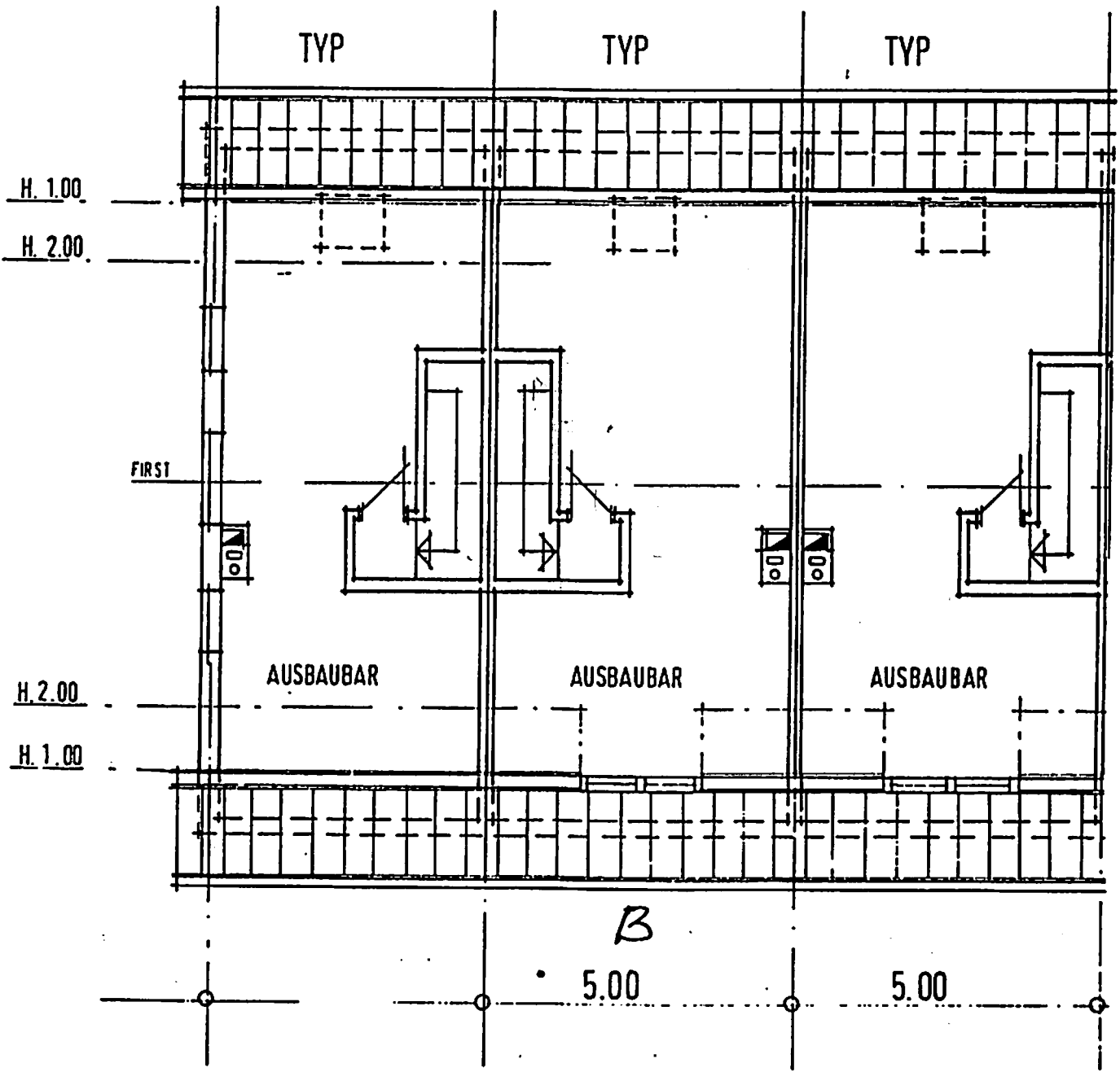
GRUNDRISS DACHGESCHOSS
