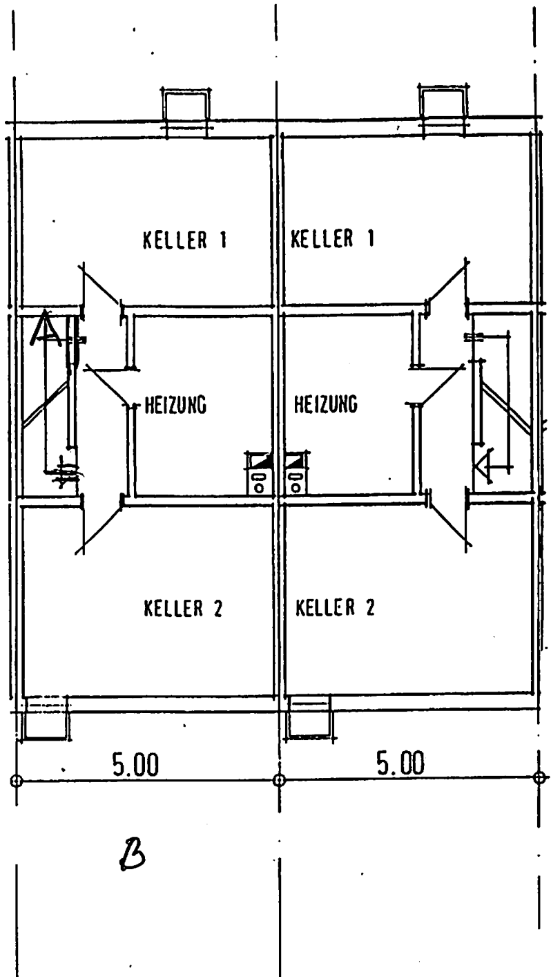
GRUNDRISS UNTERGESCHOSS
