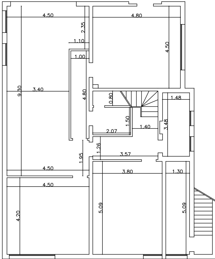
PIANTA PIANO SEMINTERRATO
