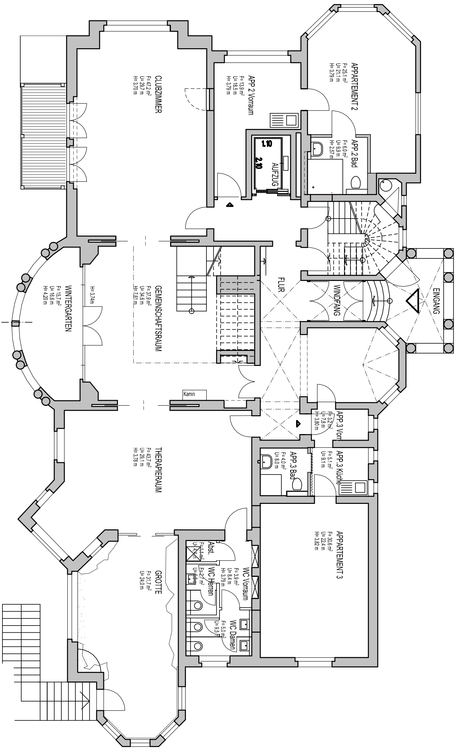
GRUNDRISS ERDGESCHOSS HAUS FELSENECK M 1: 100 Fritz- Koch - Str.11, 99817 Eisenach März 2014
