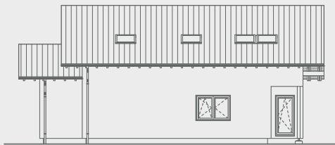
Ansicht Rechts
