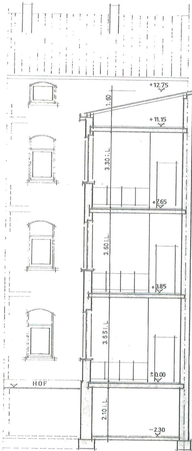
SCHNITT B-B
