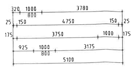
Kellergeschoss
