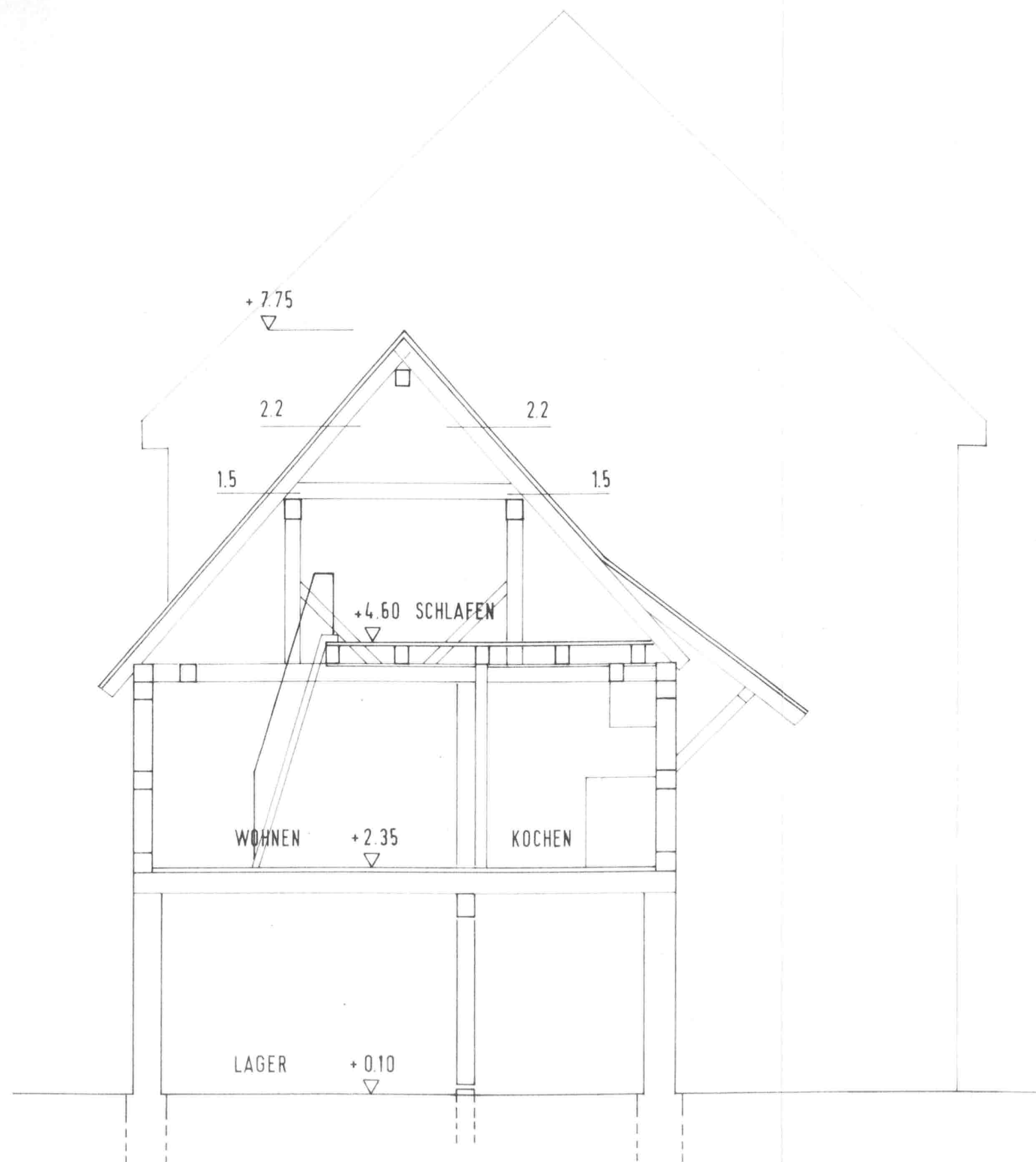
SCHNITT B-B
