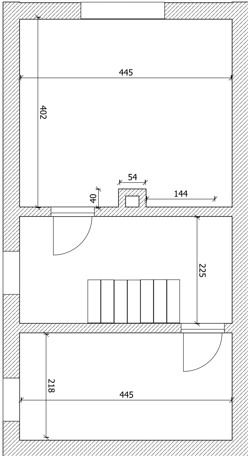
Obergeschoss Russenhäuser 11 Bernstadt/ OT Russen
