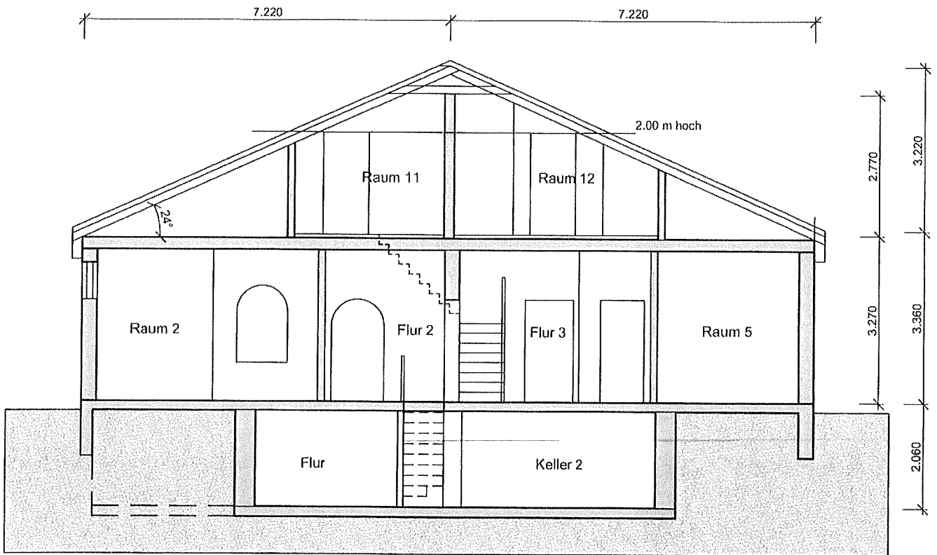
Schnitt A-A
