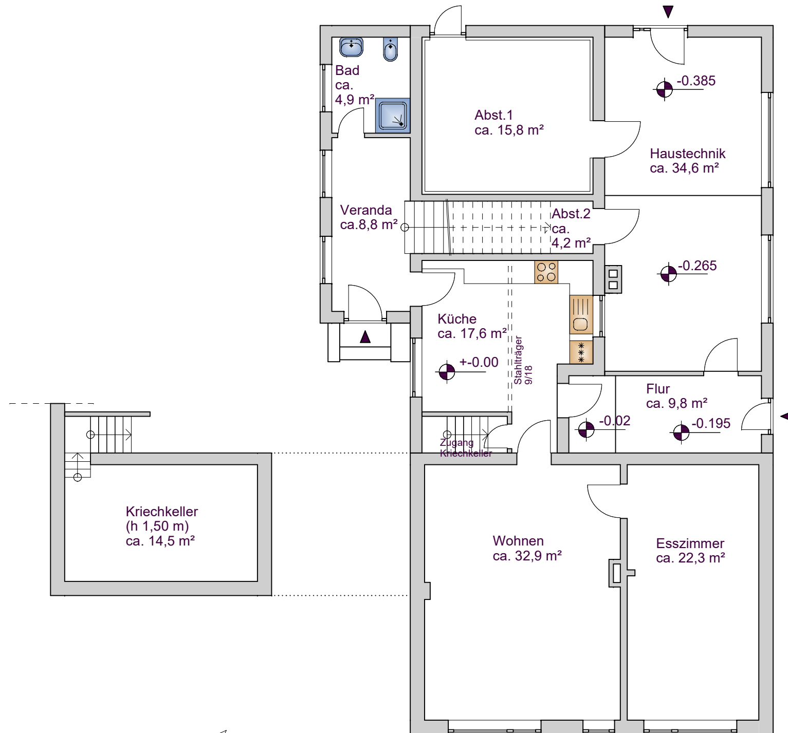
Erdgeschoss
