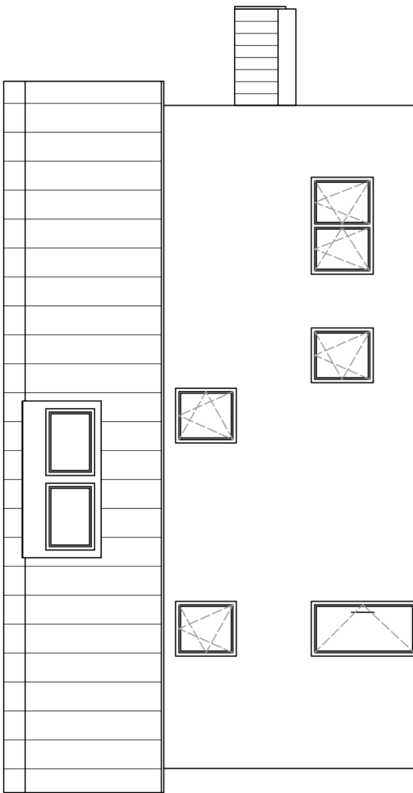
Ansicht Westen
