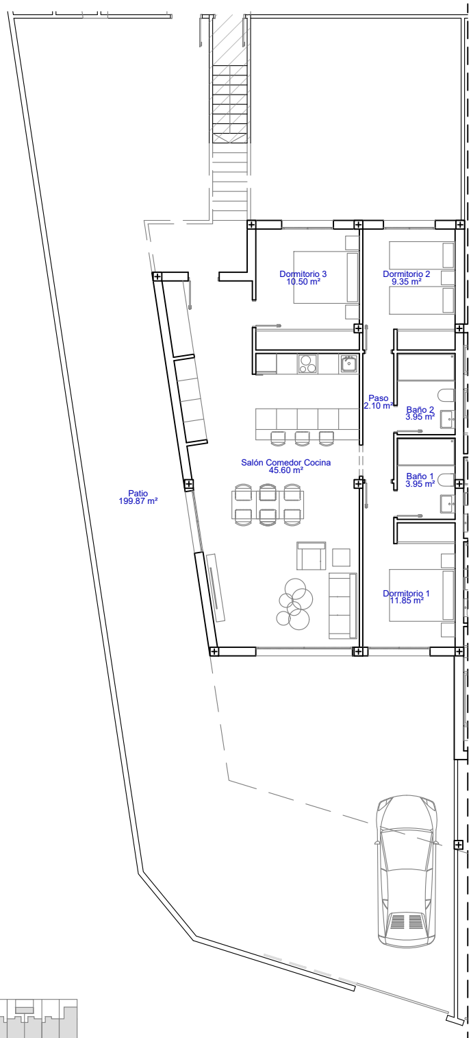
Planta Baja E:1/150
