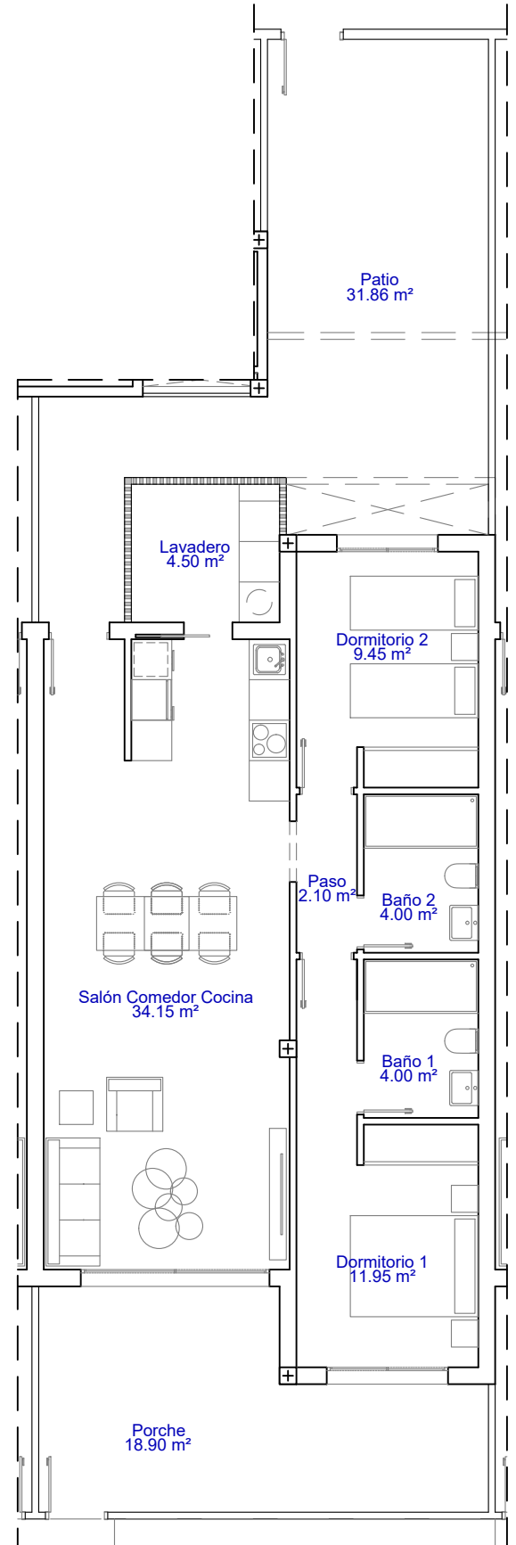
Planta Baja E:1/100
