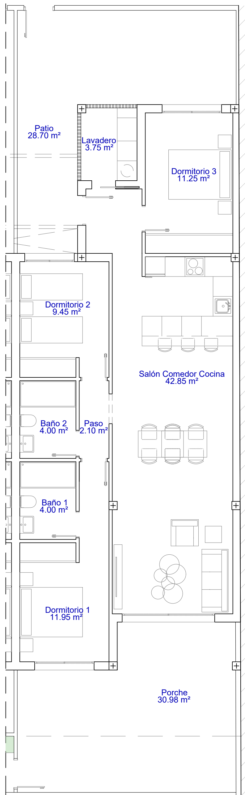
Planta Baja E:1/100
