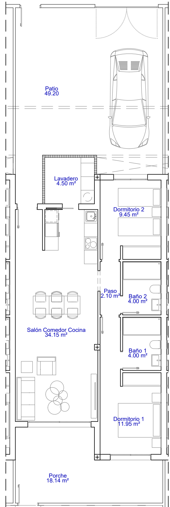
Planta Baja E:1/100
