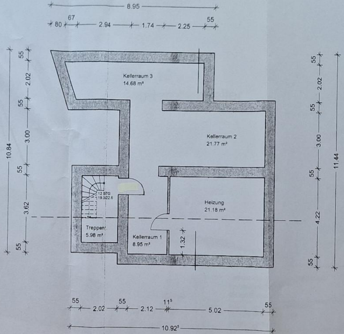
Grundriss Keller
