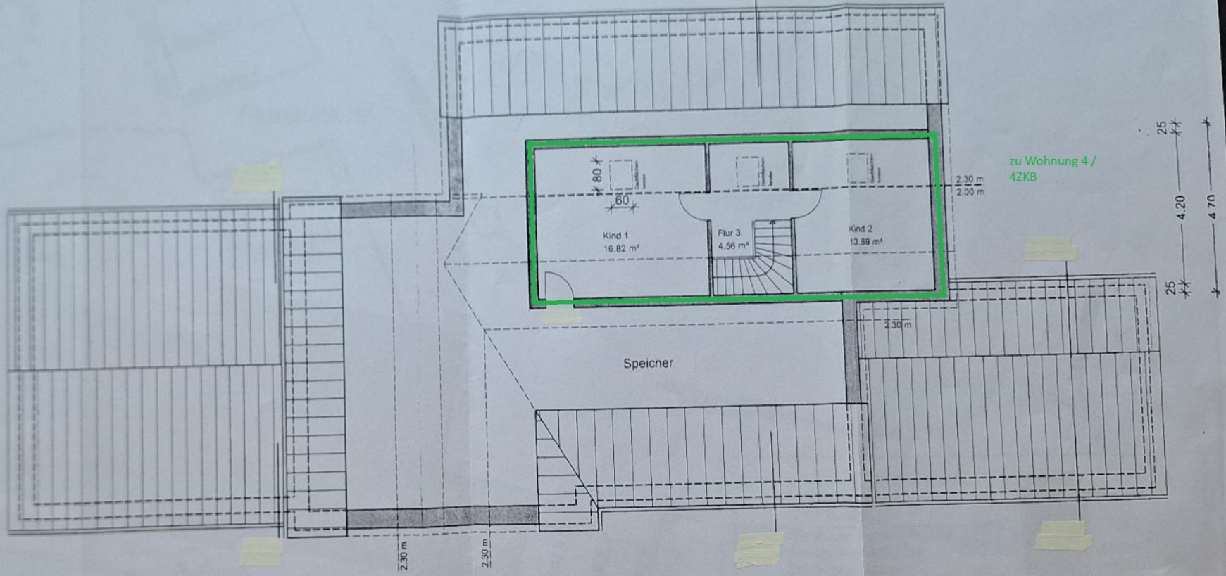
Grundriss Dachgeschoss
