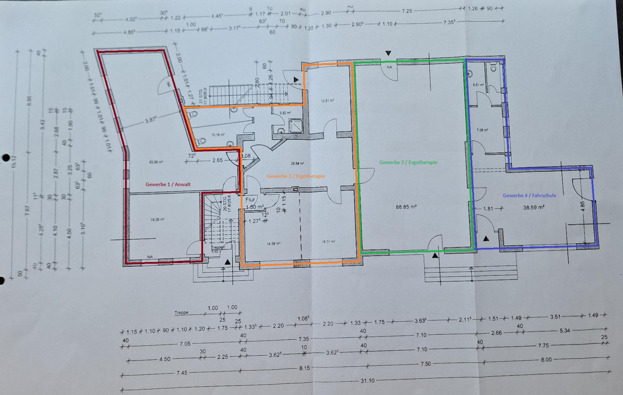
Grundriss Erdgeschoss
