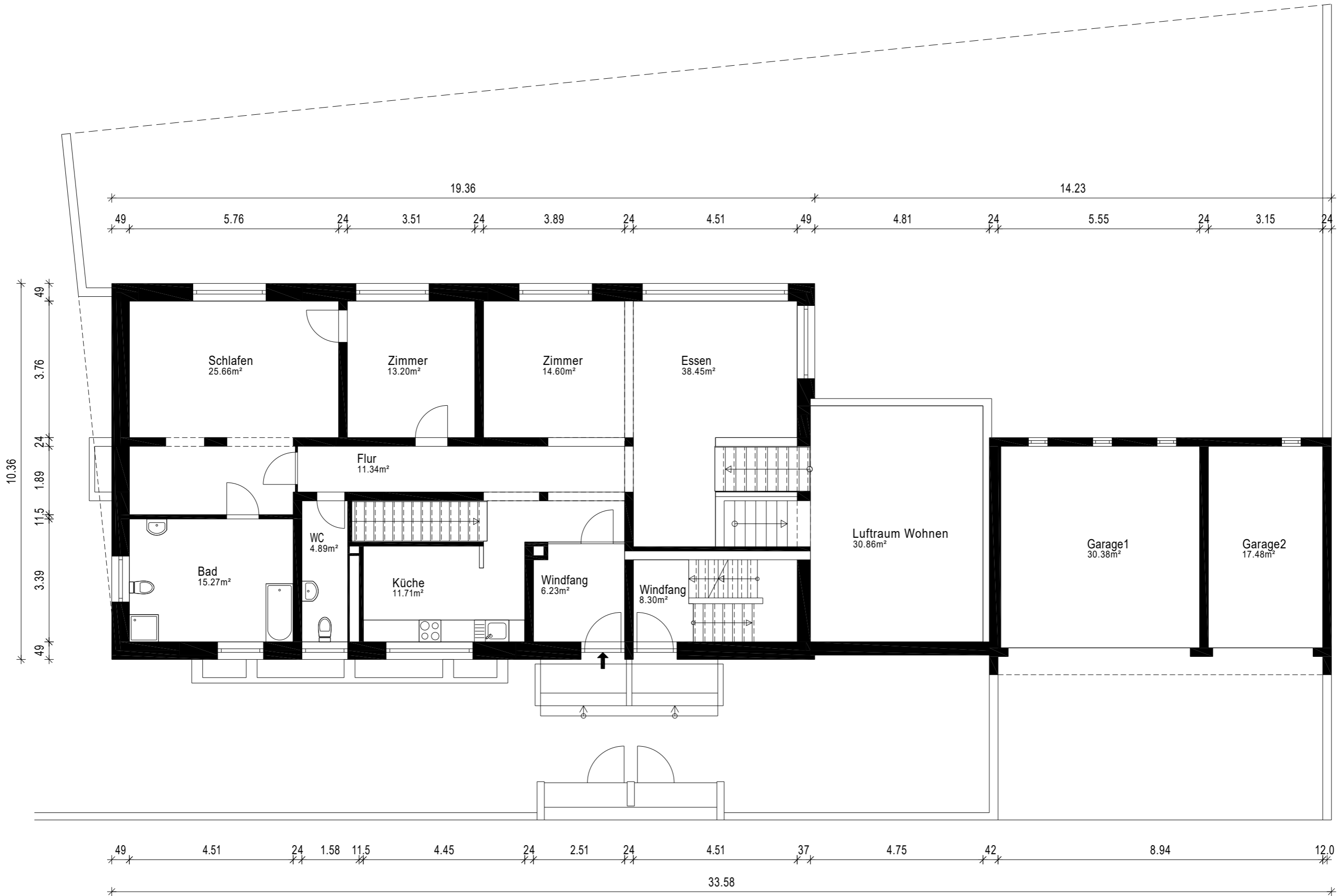
Erdgeschoss
