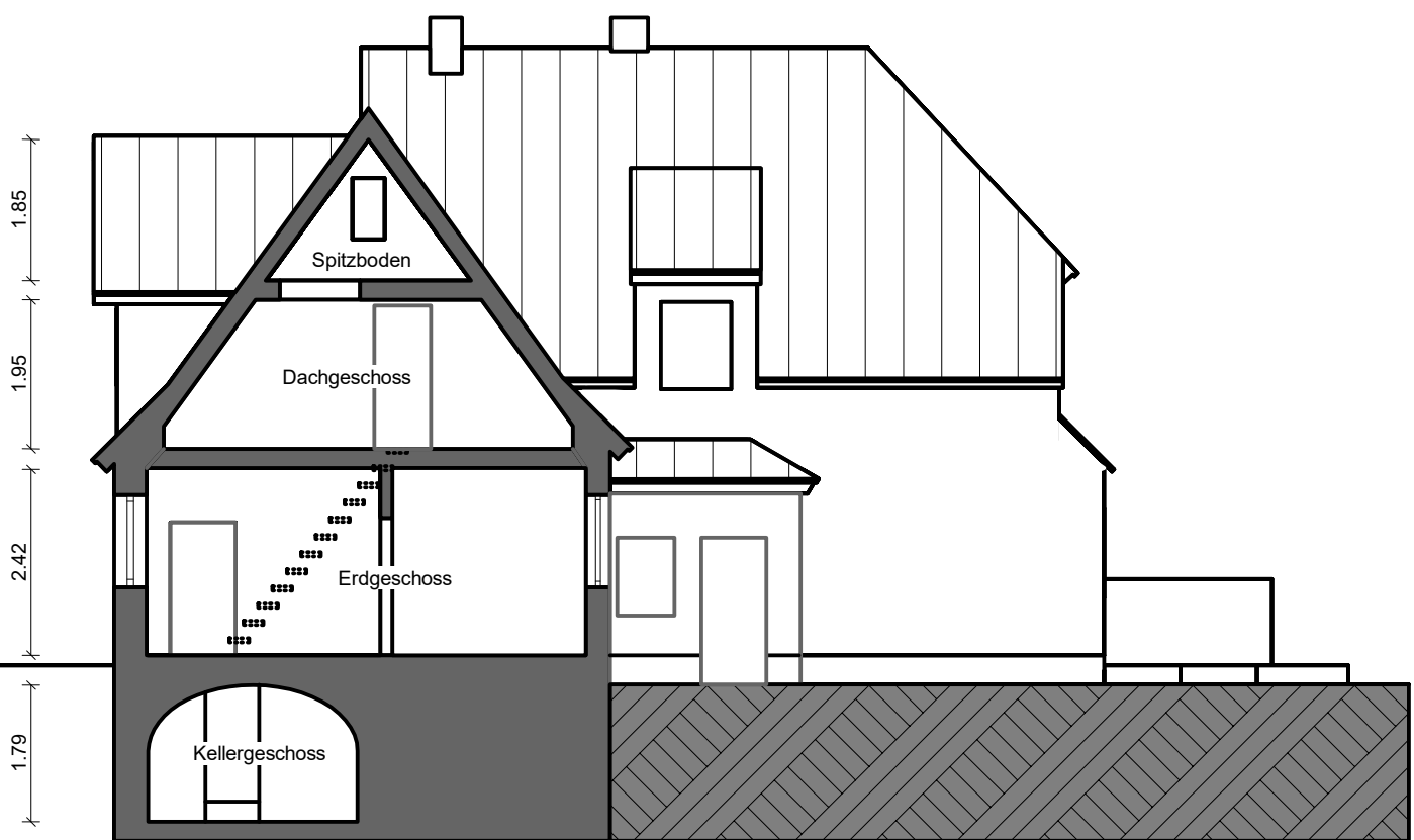
Schnitt A-A
