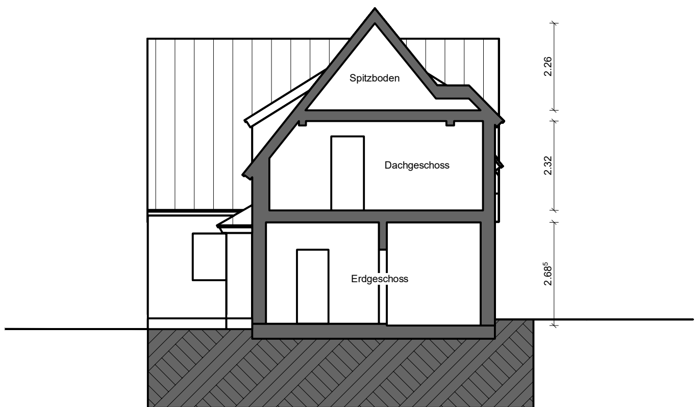
Schnitt B-B
