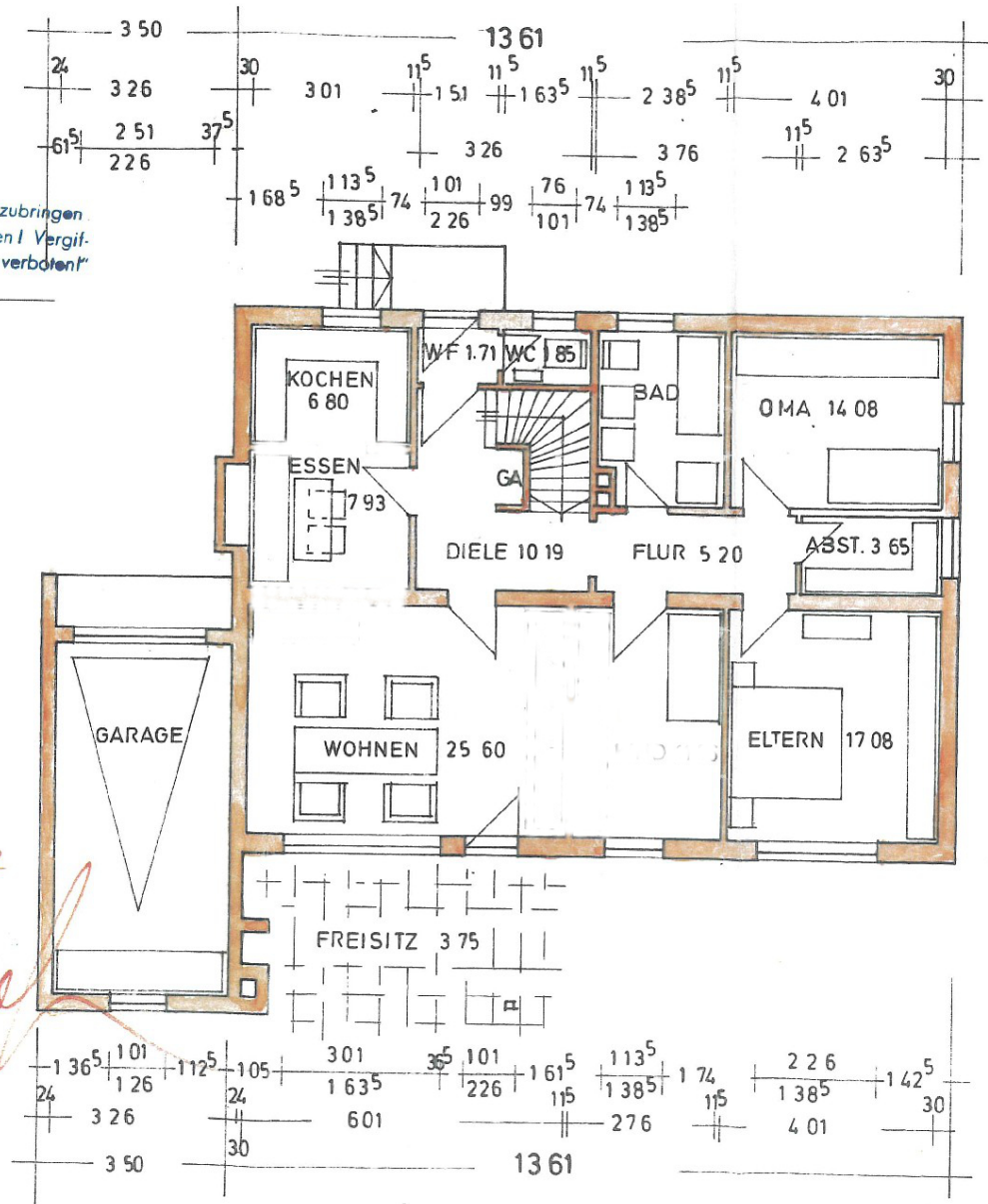
ERDGESCHOSS
