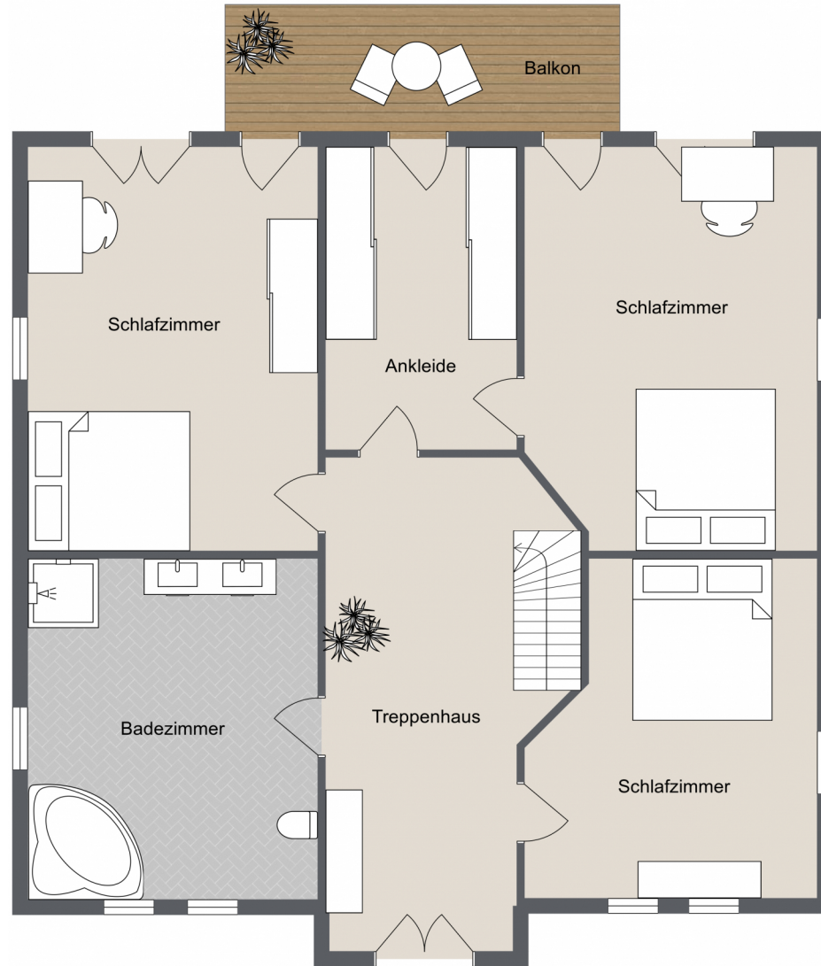
Obergeschoss
