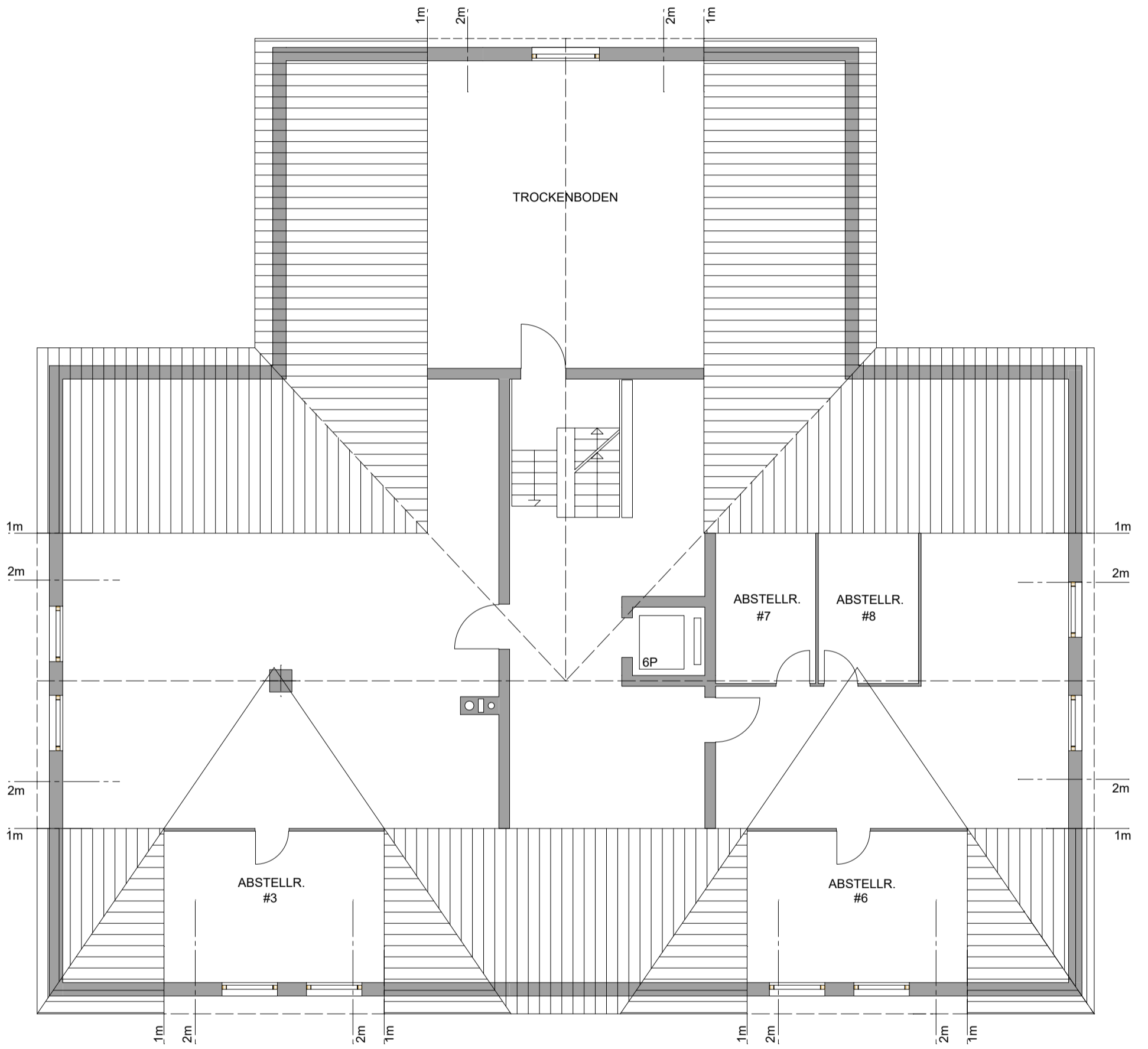
SPITZBODEN
