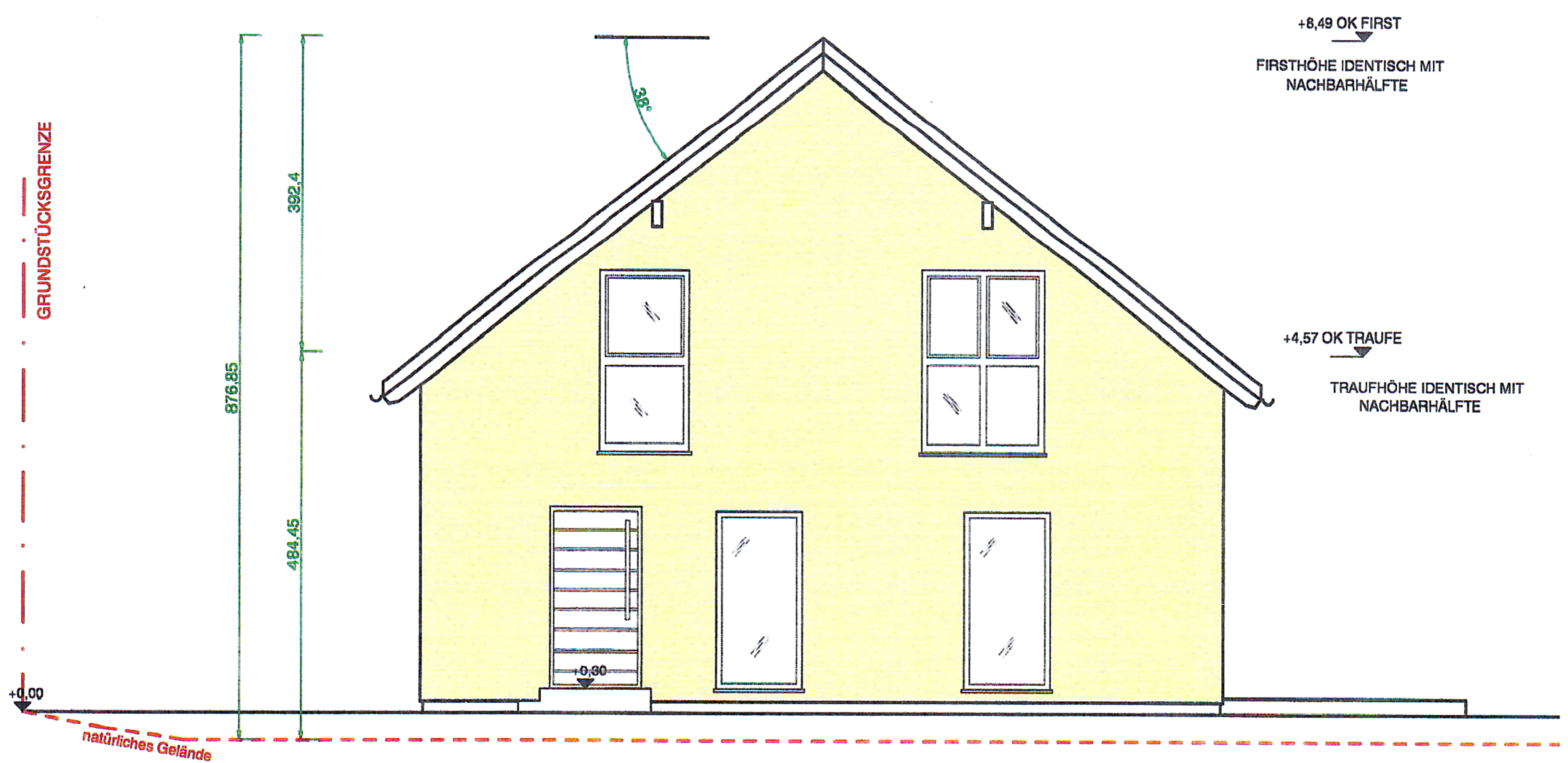
WESTANSICHT m 1:100
