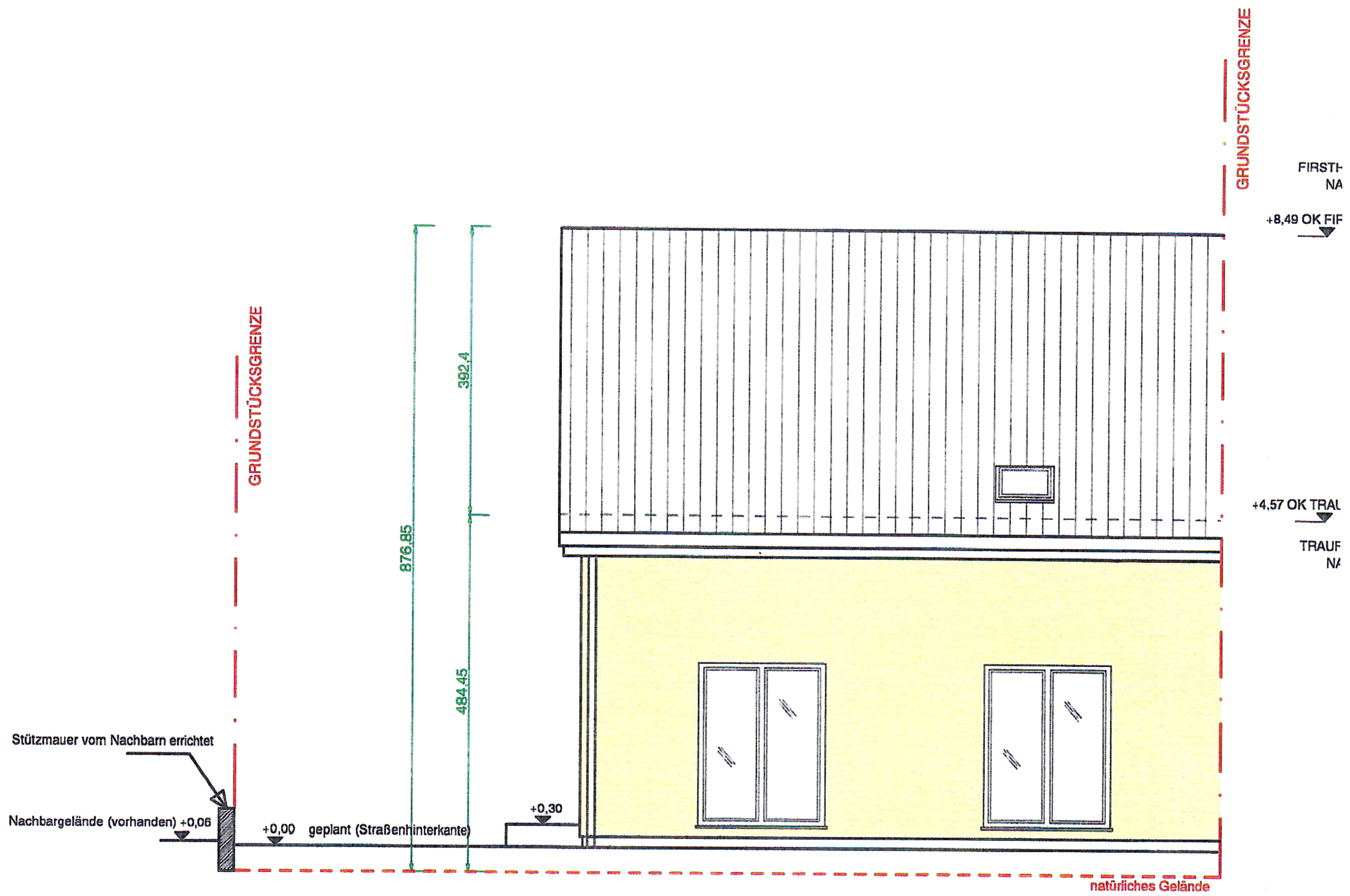
SÜDANSICHT m 1:100
