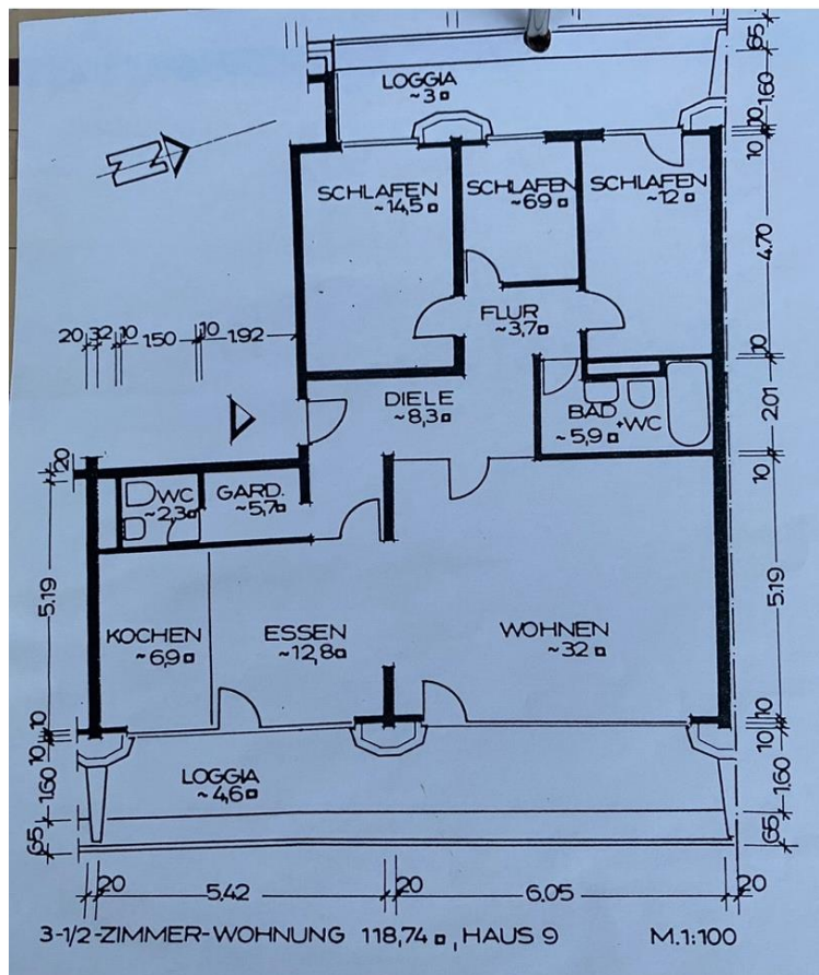
Grundriss
