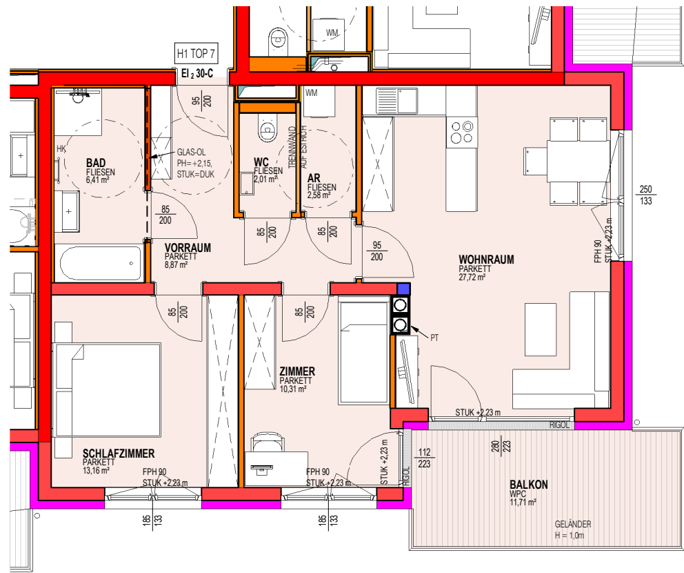
1. OBERGESCHOSS M 1 : 100
