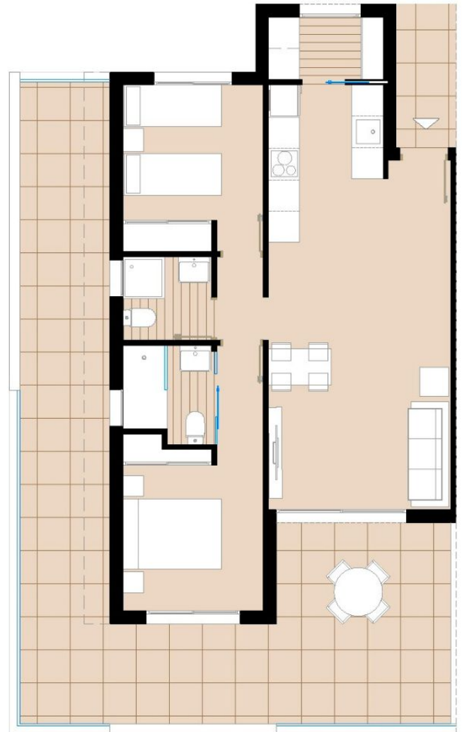
First Floor/ Planta Primera (E:1/100)
