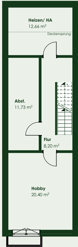
KELLERGECHOSS
