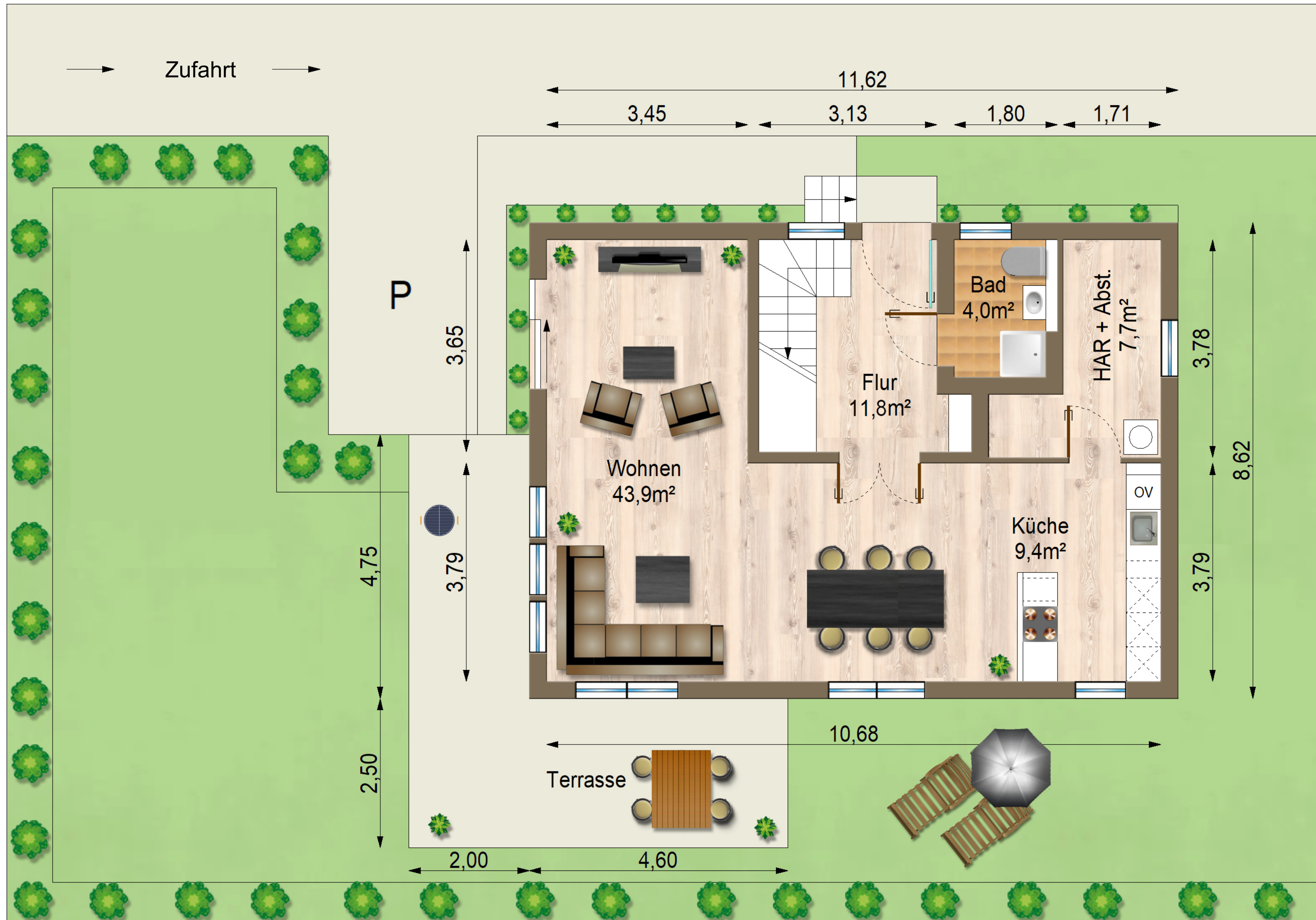
Erdgeschoss
