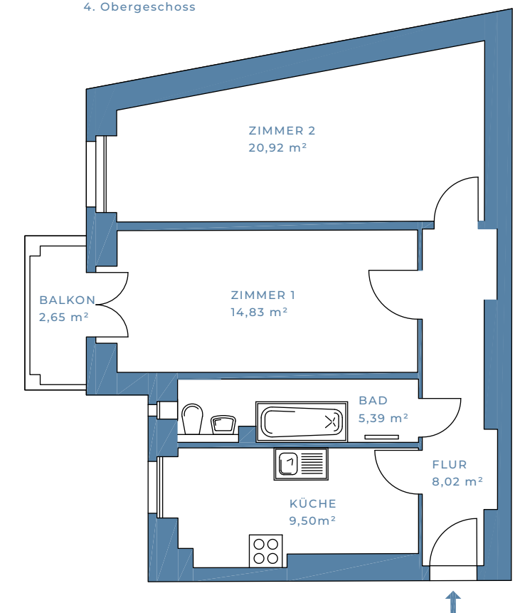
4. Obergeschoss
