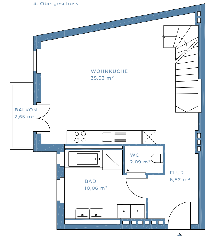
4. Obergeschoss
