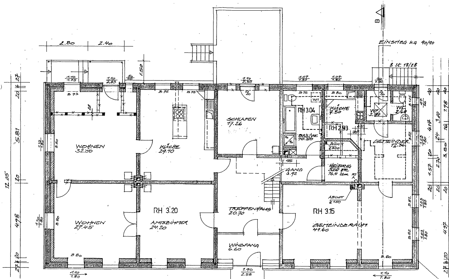
ERDGESCHOSS
