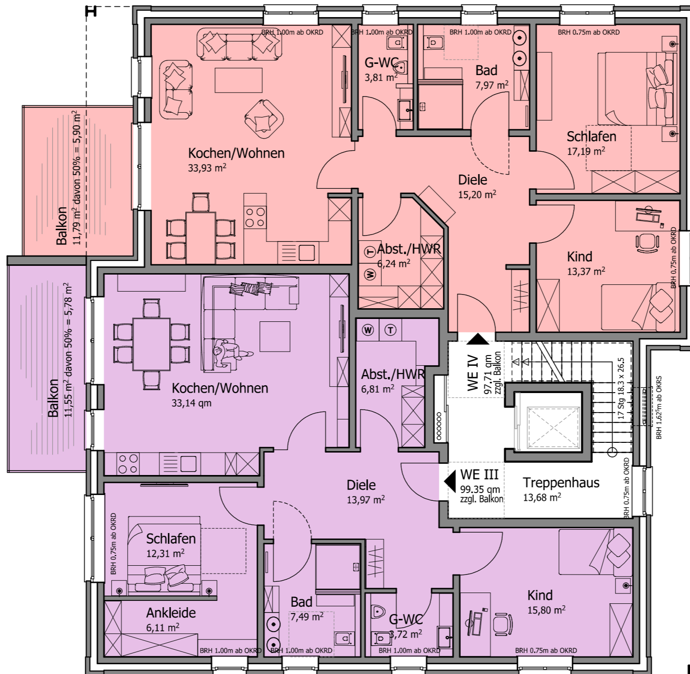
GRUNDRISS OBERGESCHOSS
