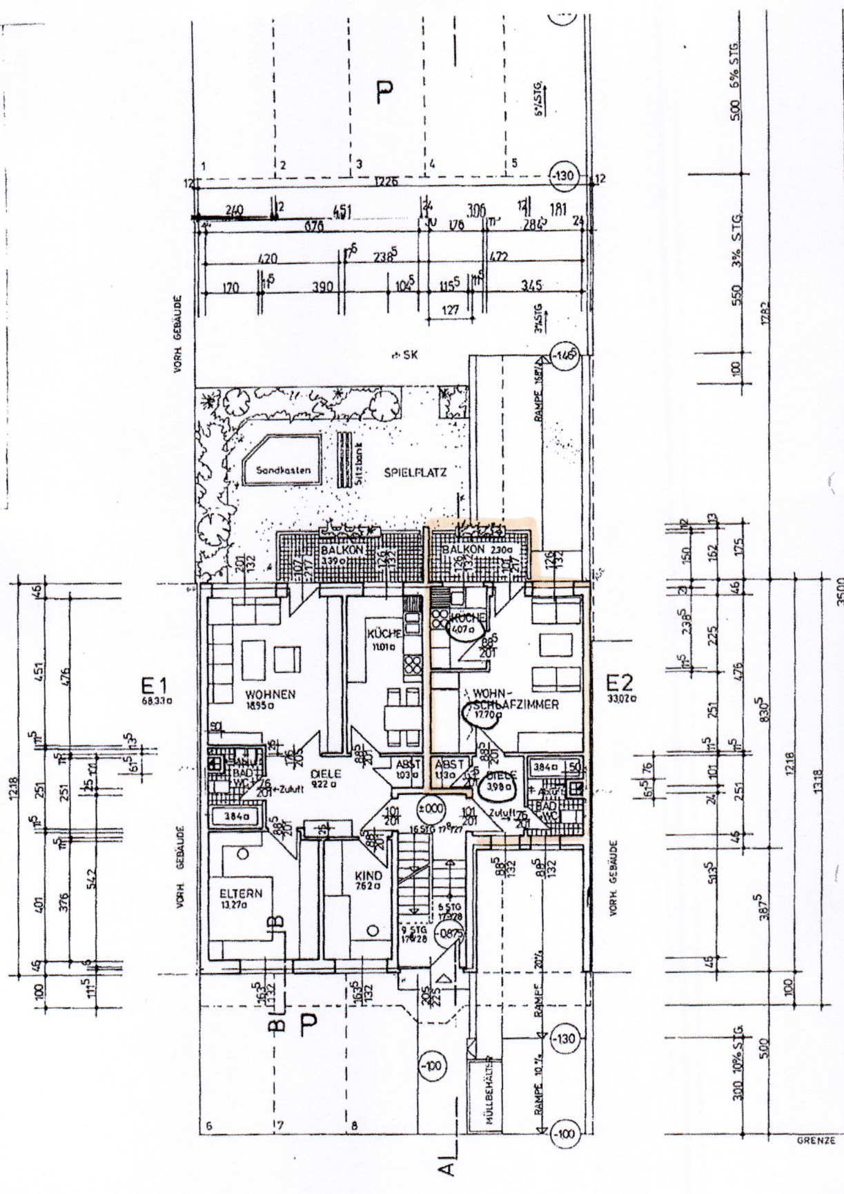
ERDGESCHOSS MASSTAB 1:100
