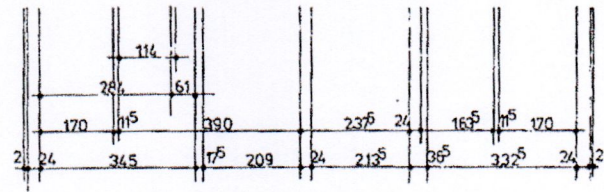
ERDGESCHOSS MASSTAB 1:100
