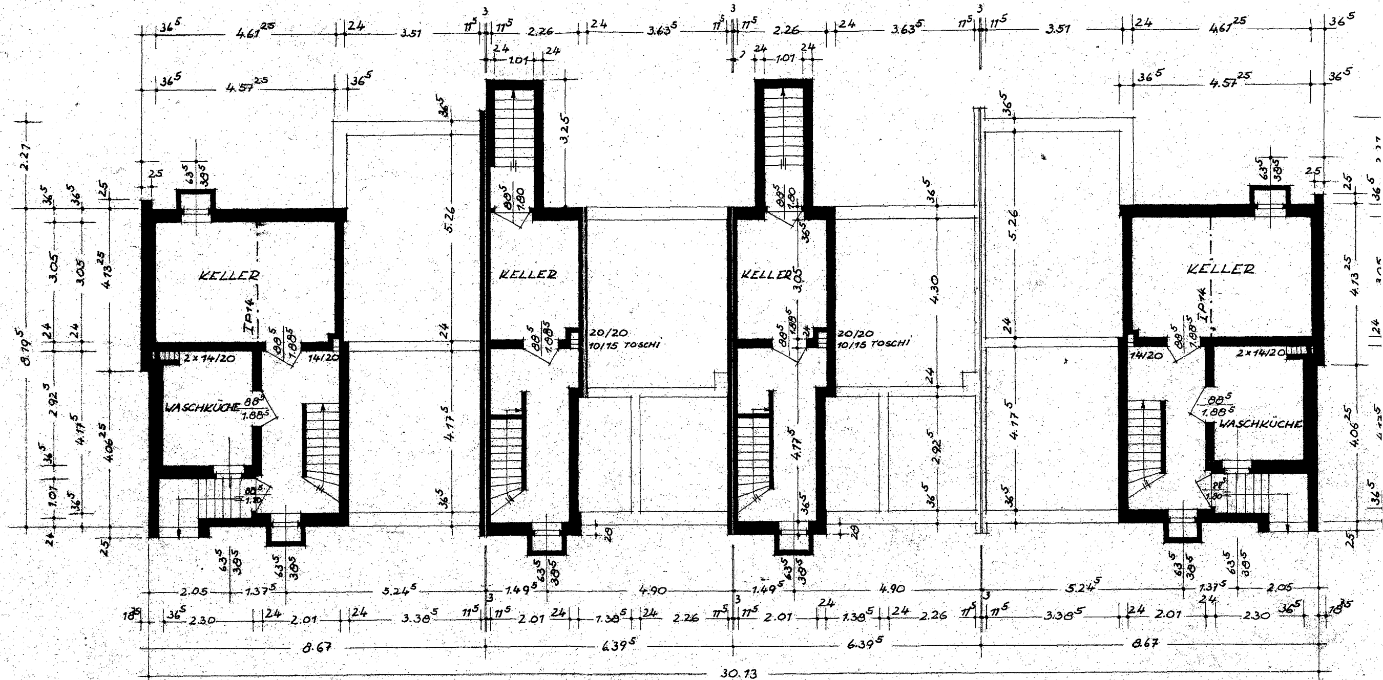
KELLERGESCHOSS - GRUNDRISS
