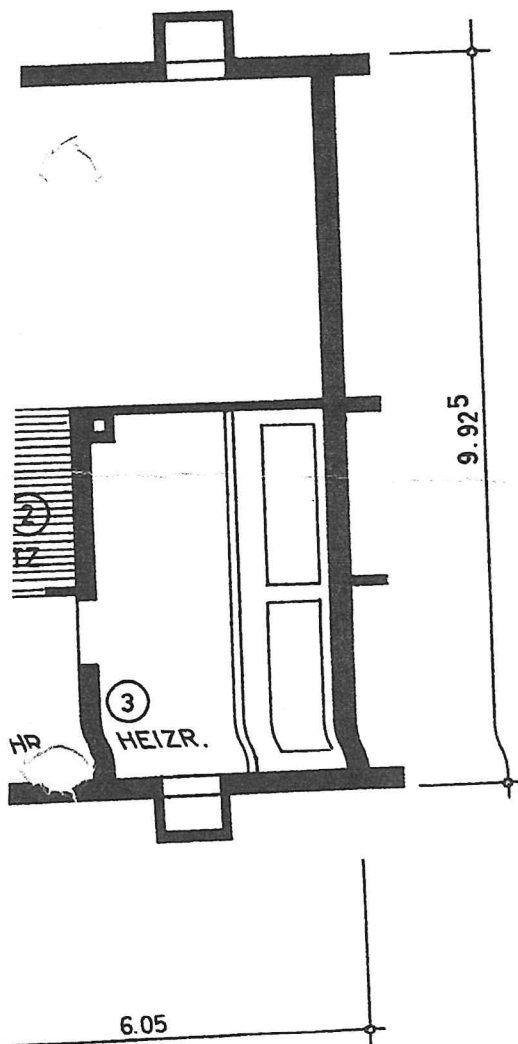
ERGESCHOSS
