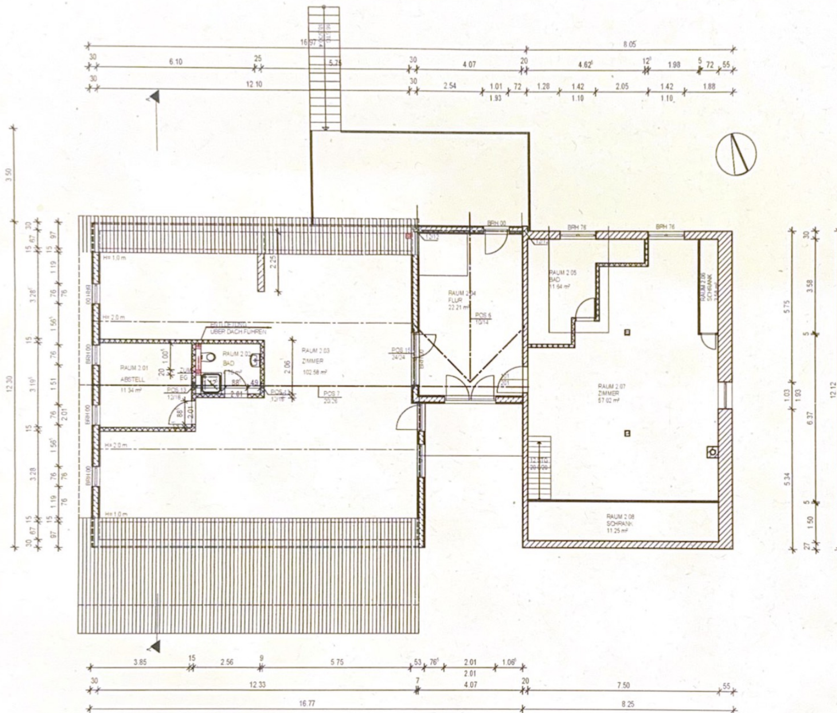
GRUNDRISS DACHGESCHOSS
