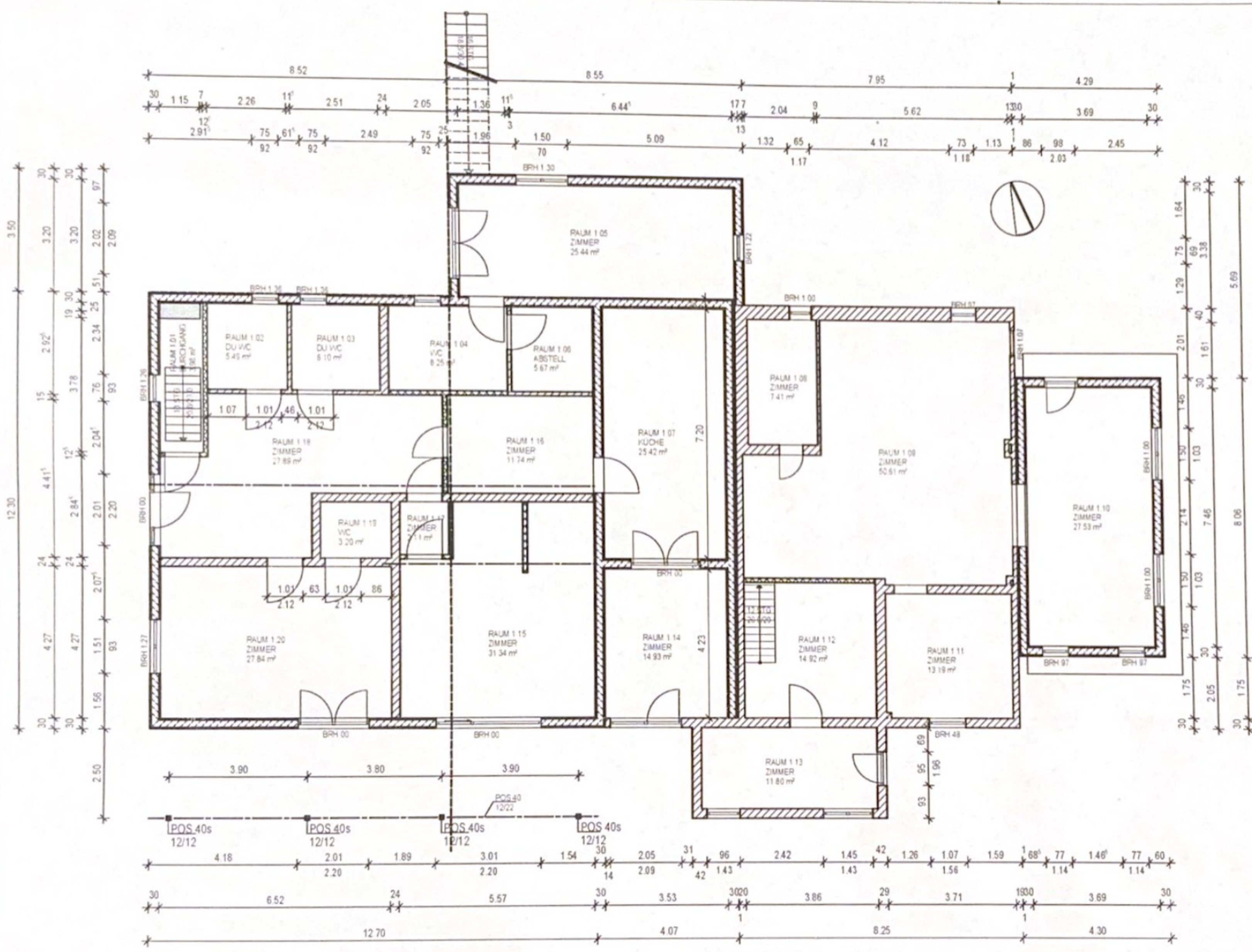
GRUNDRISS ERDGESCHOSS
