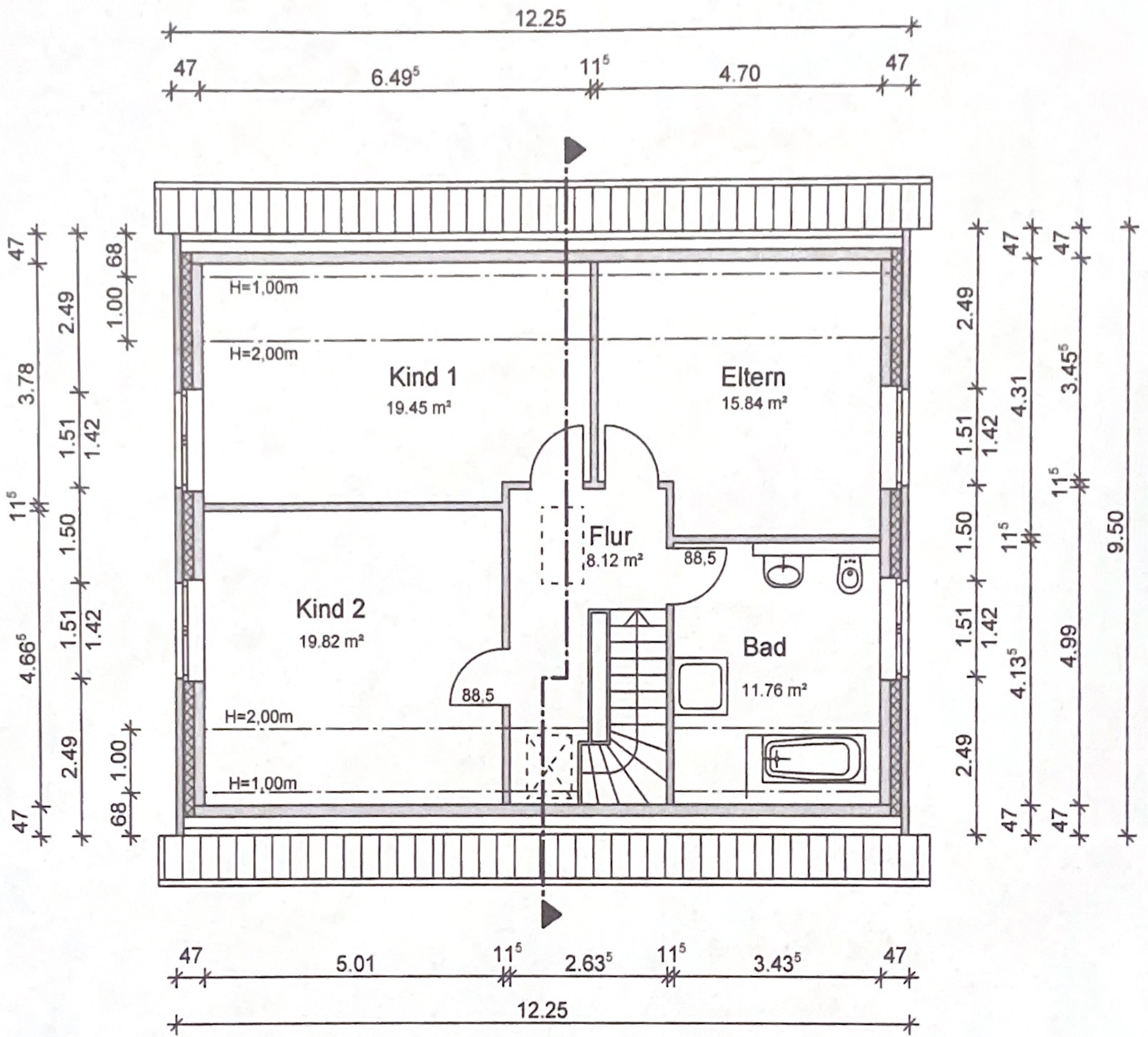
Dachgeschoss
