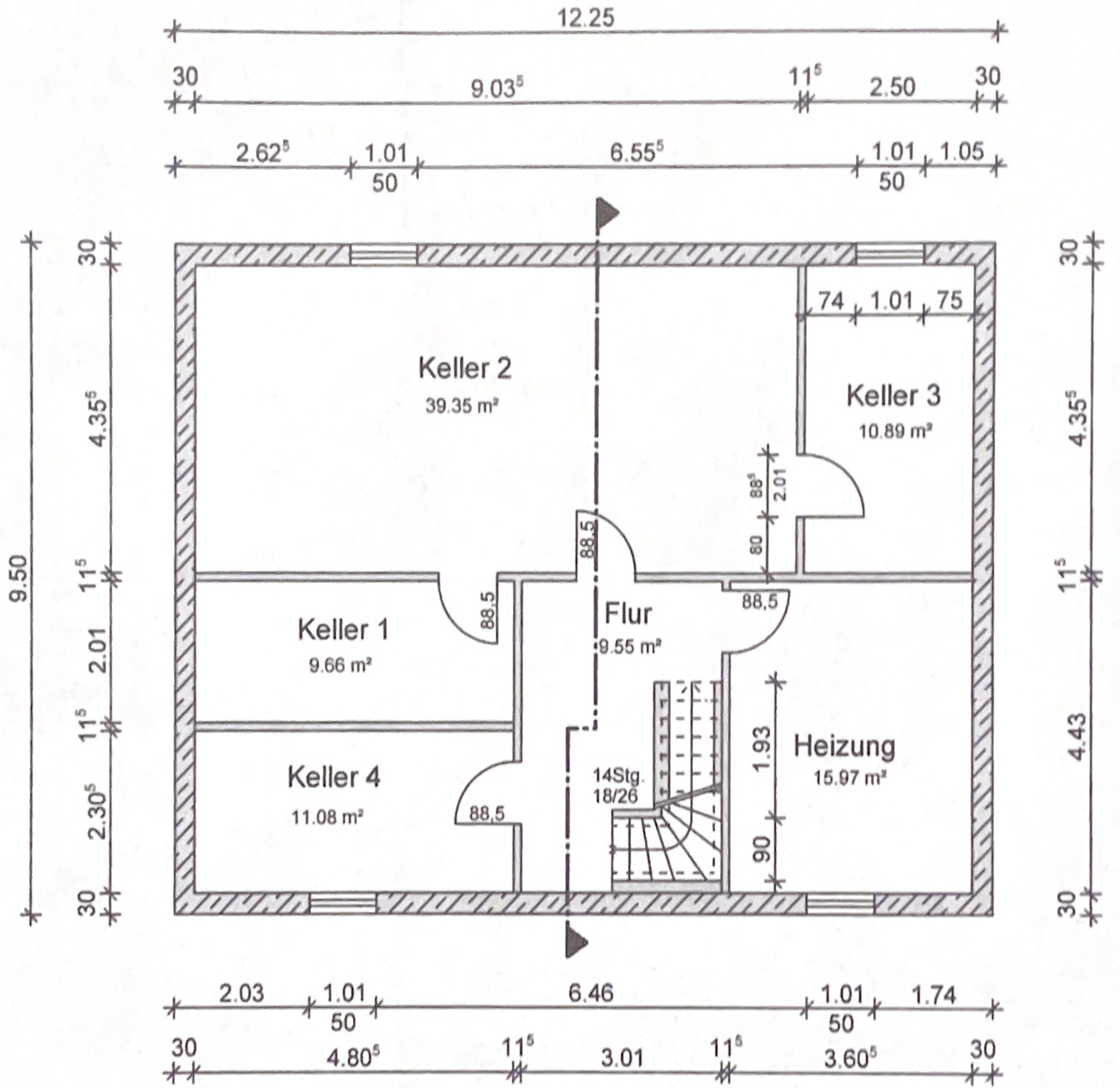
Kellergeschoss
