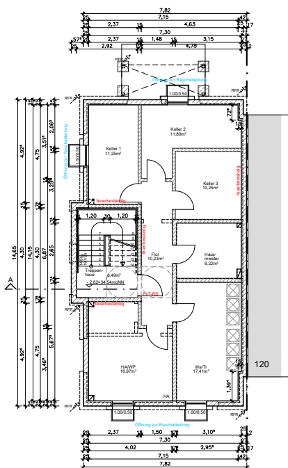
Kellergeschoss
