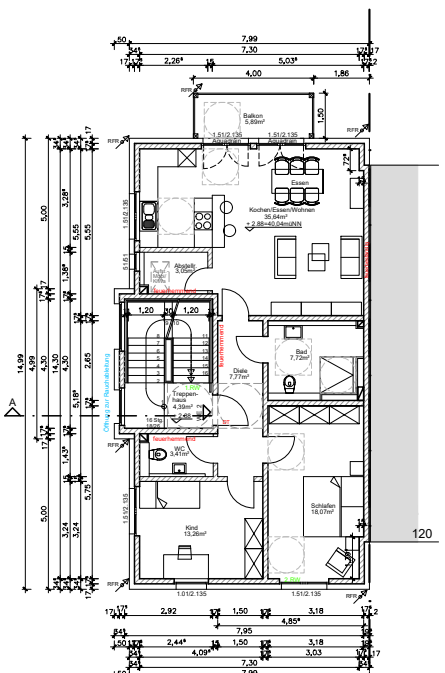
Obergeschoss
