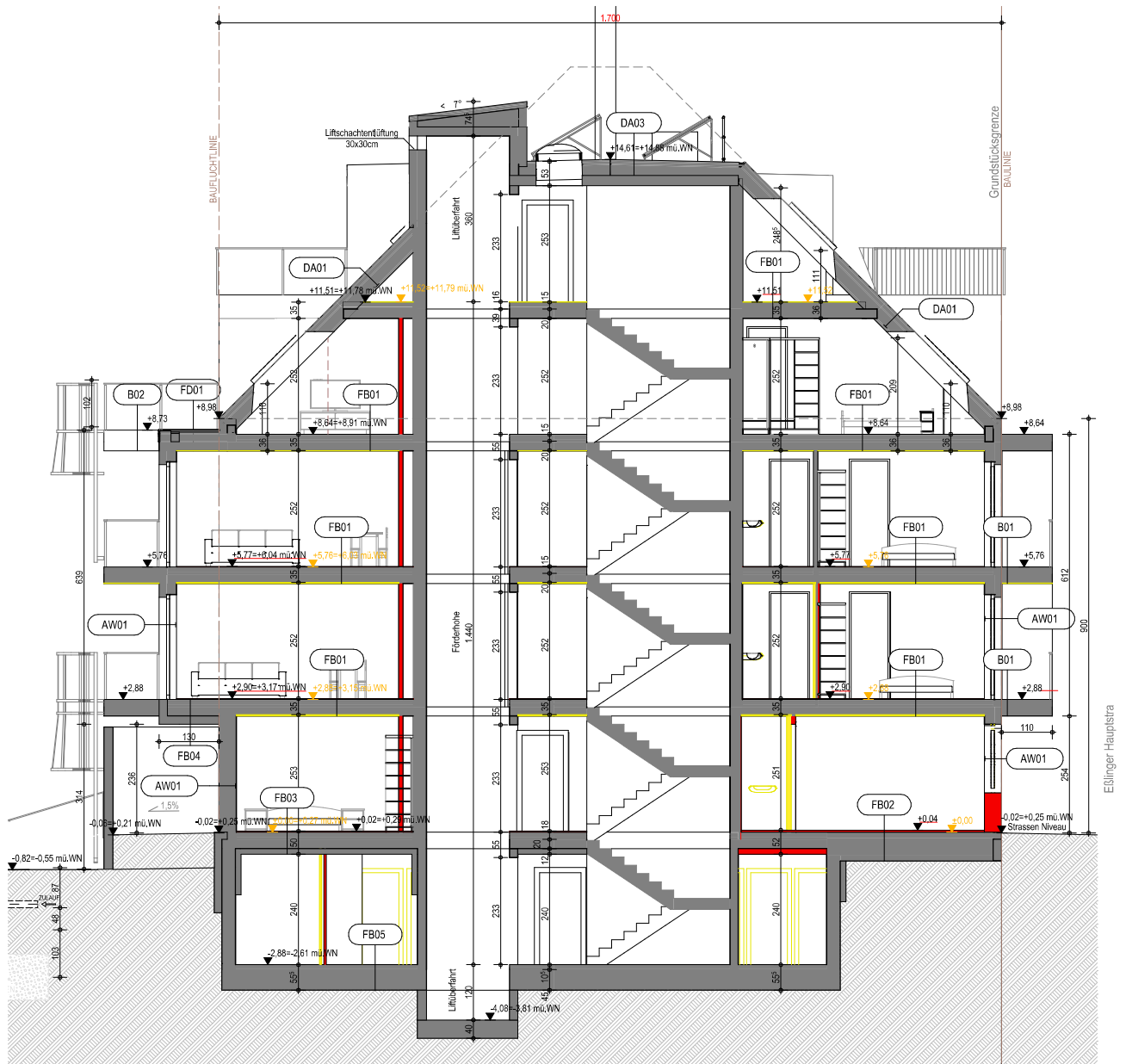
SCHNITT A
