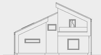
Ansicht Hinten
